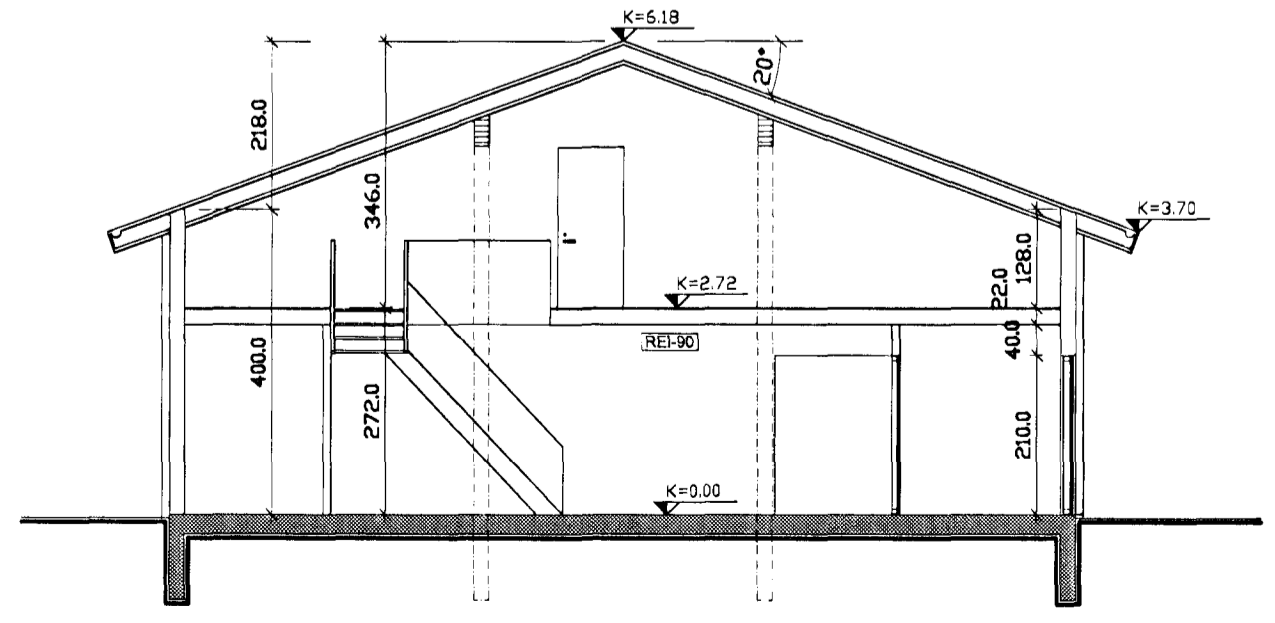
Snið A-A 1:100
