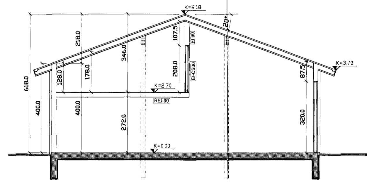
Snið B-B 1:100
