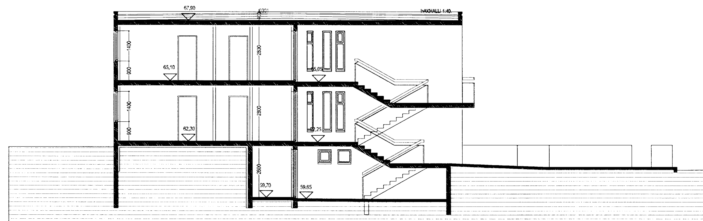
SNÍÐ B-B. MKV. 1:100.
