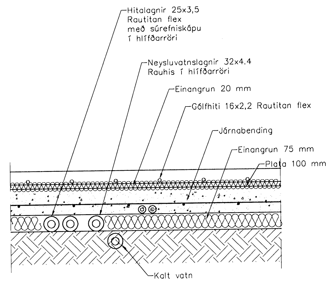
Hitla- og Neysluvotnslagðir. Snið í botnplötu, 1:10
