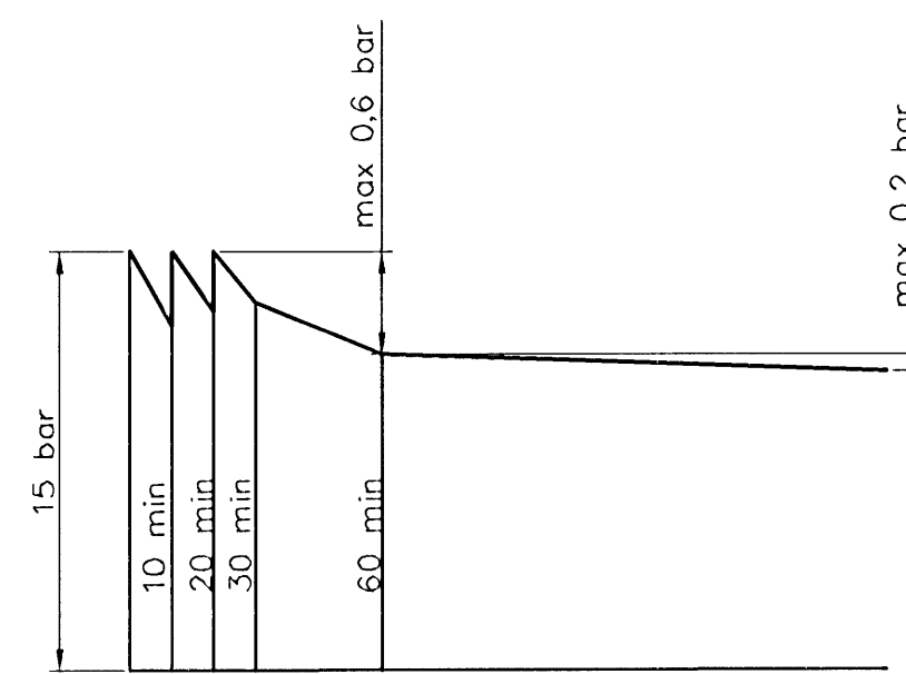
Þrjústípröfun á neysluvatnslögnum línurit
