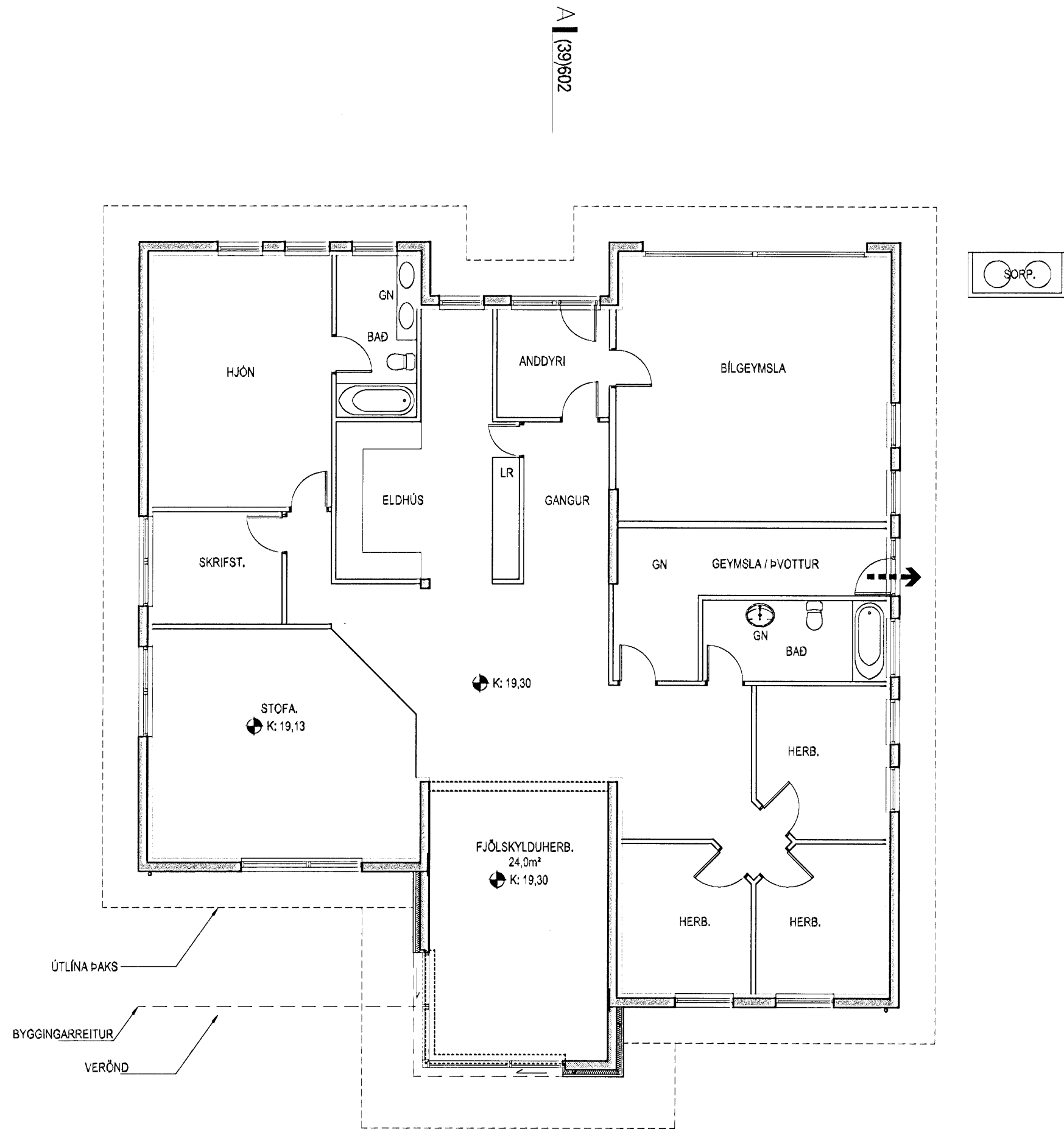
GRUNNMYND MKV 1:100
