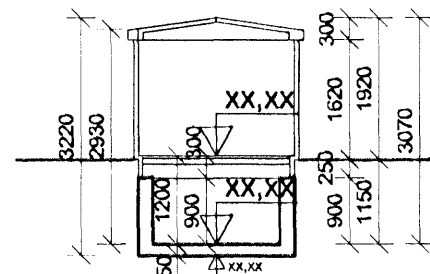
Snið A-A
