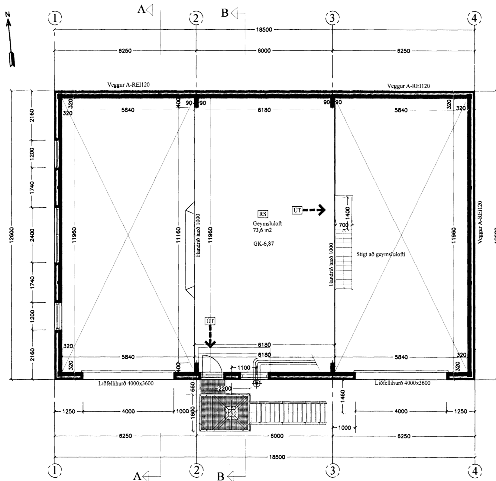
GRUNNMYND AF MILLILOFTI MKV.2
