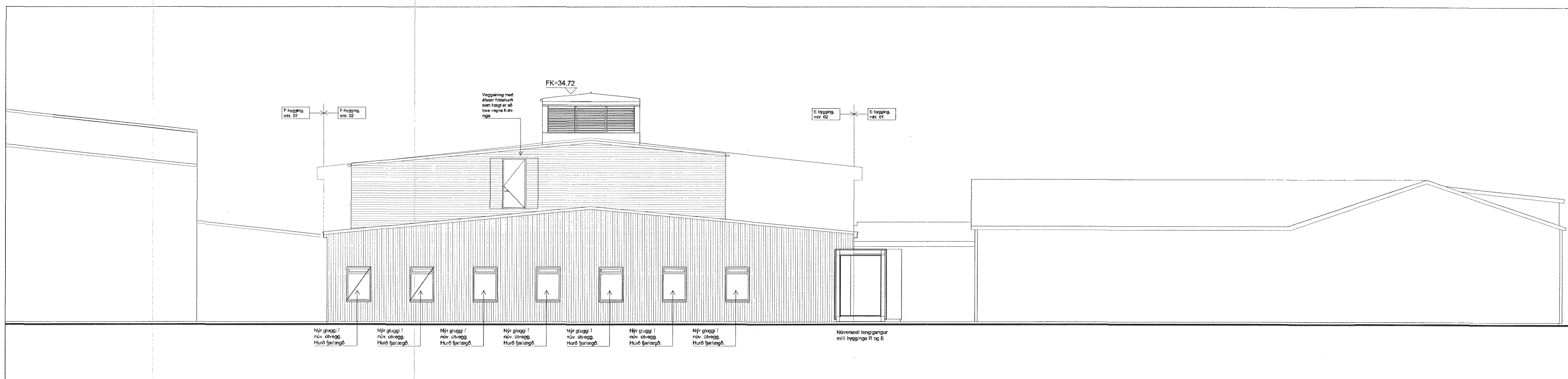
ÚTLIT NORÐUR, 1:100
