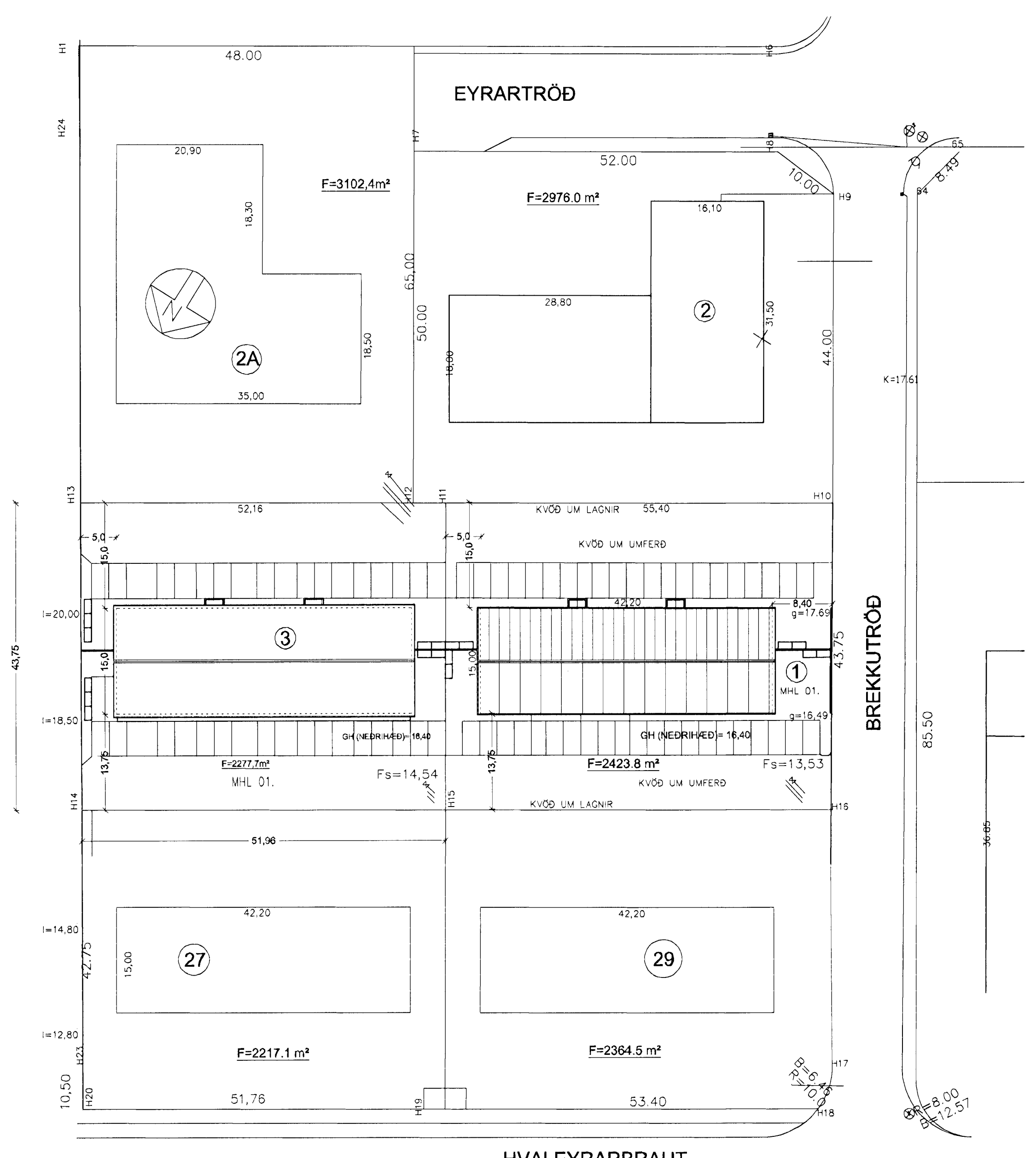
AFSTÖÐUMYND MKV. 1: 500.
