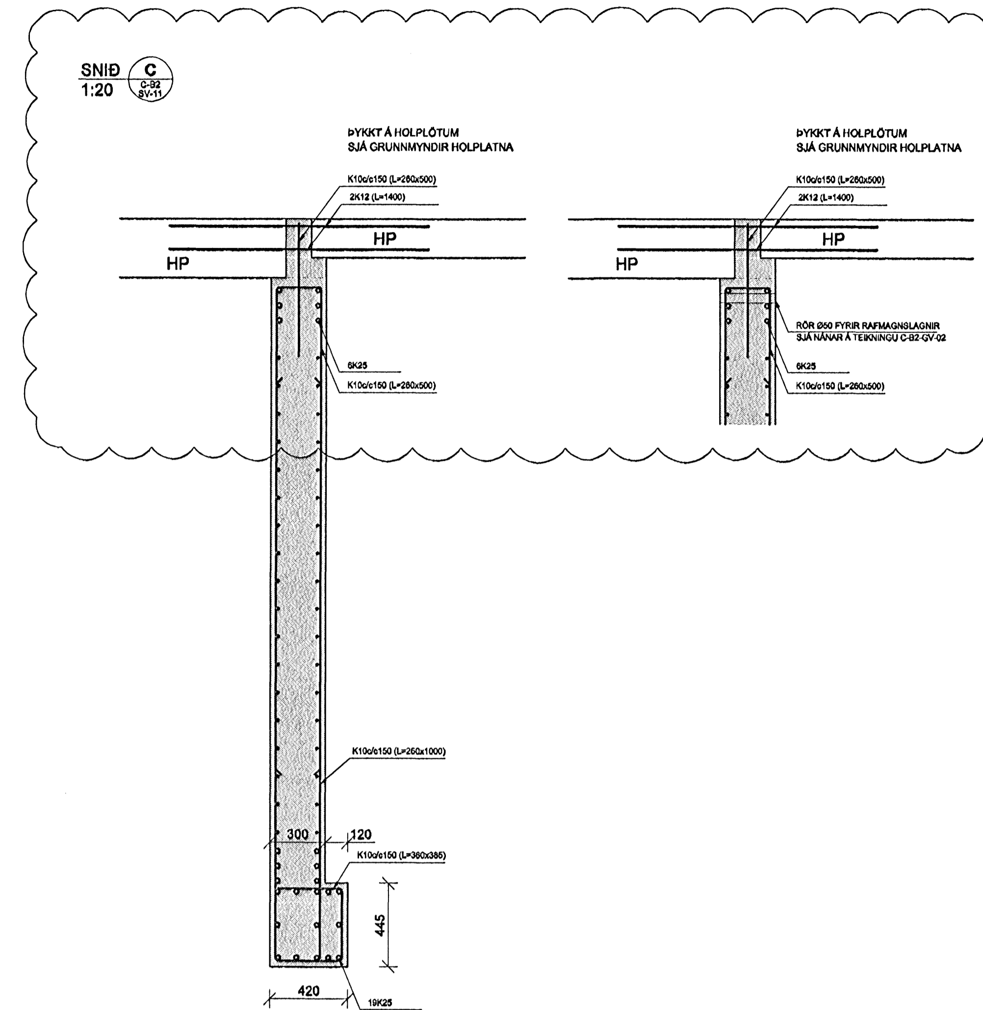
SNID D 1:20 S-52 01-11
