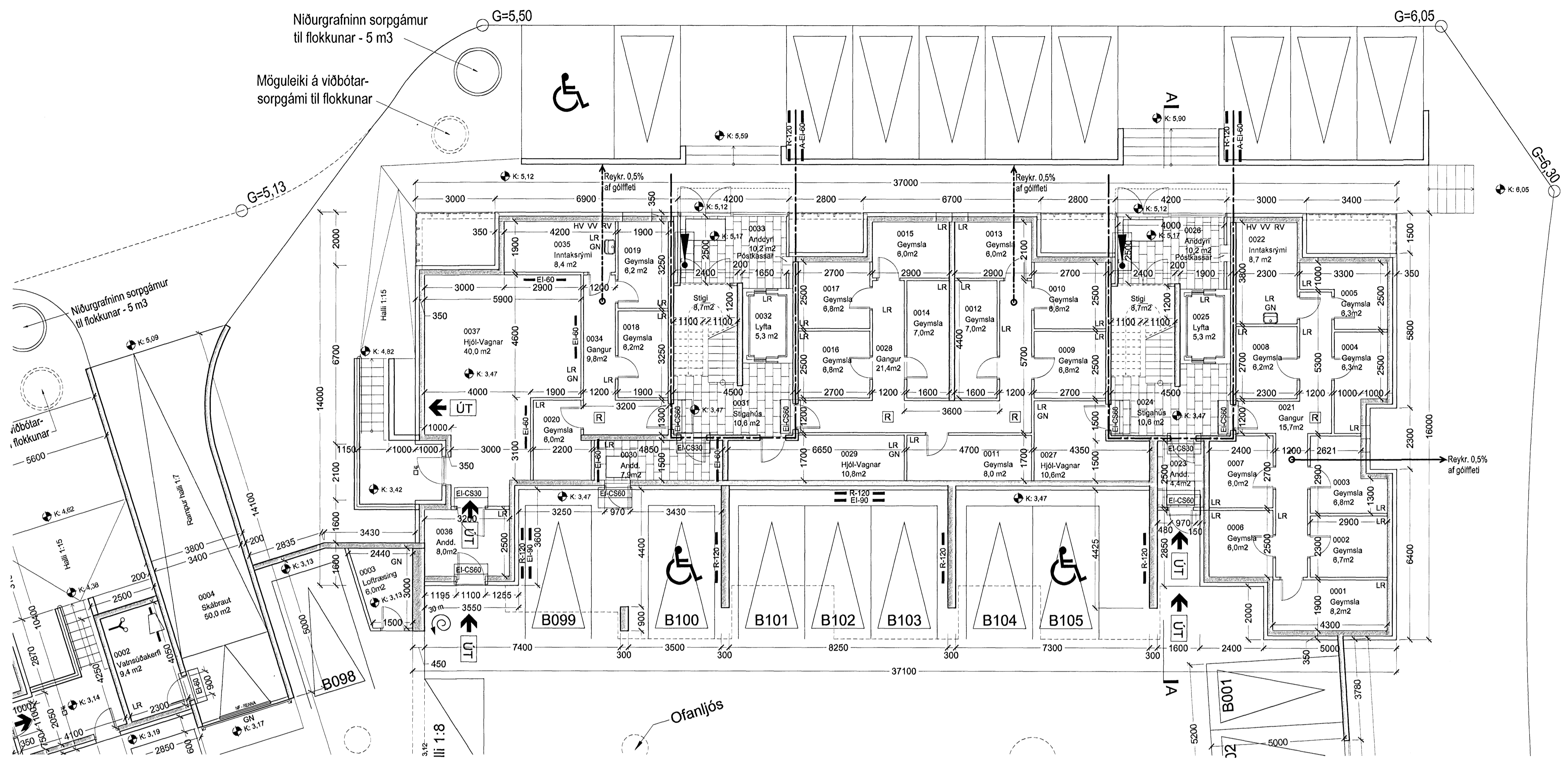
Grunnmynd kjallara i mkv. 1:100
