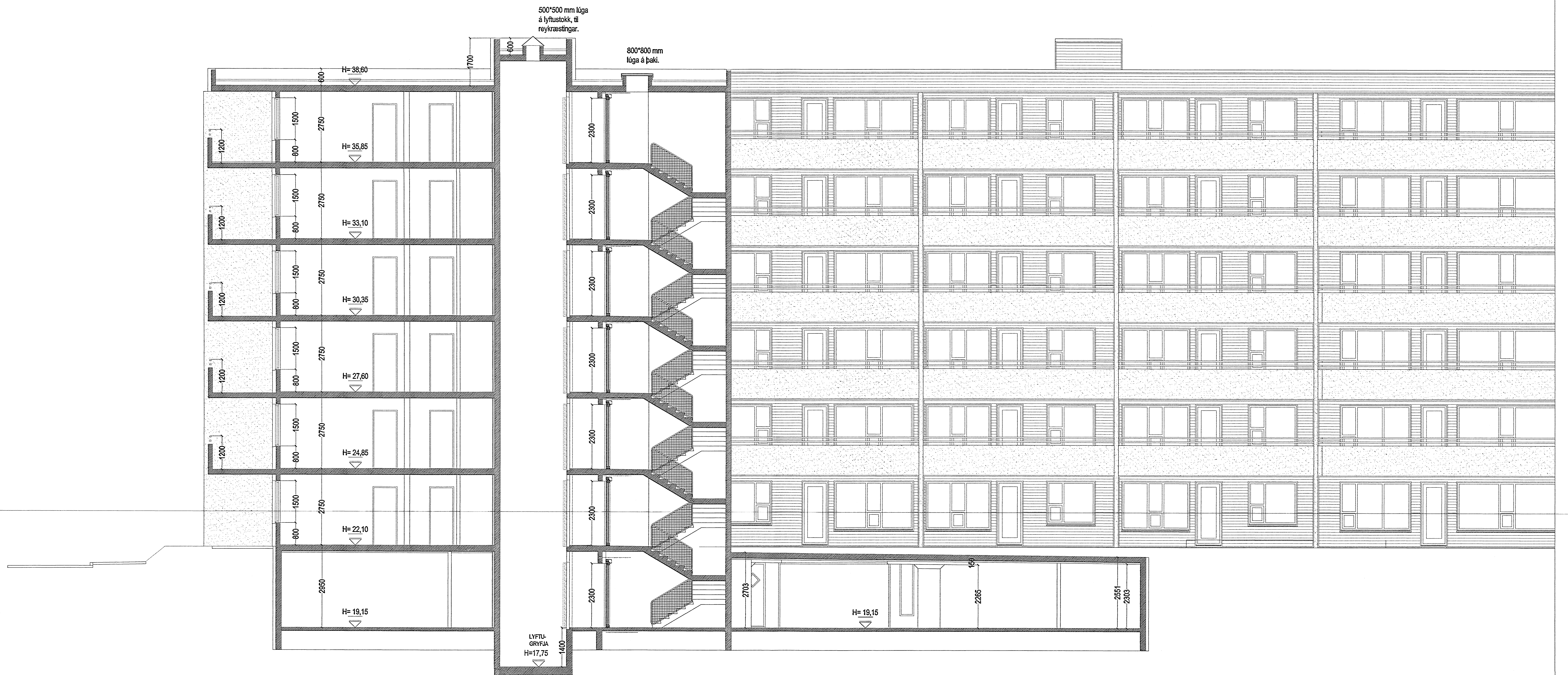
SNID B-B. MKV. 1:50.
