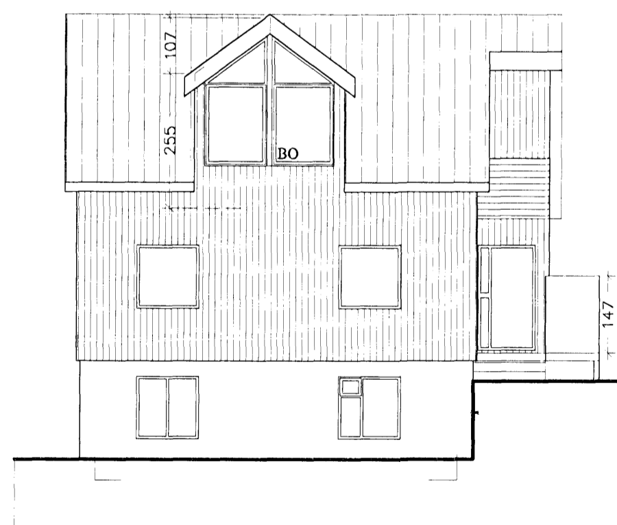
ÚTLIT VESTUR 1:100
