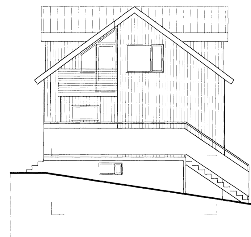
ÚTLIT SUÐUR 1:100
