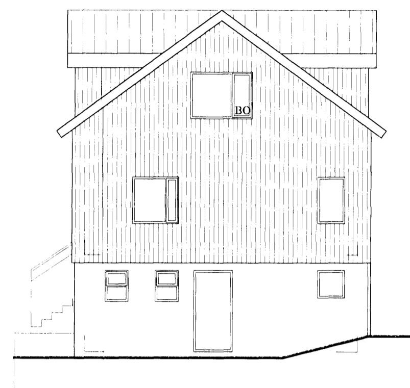
ÚTLIT NORÐUR 1:100
