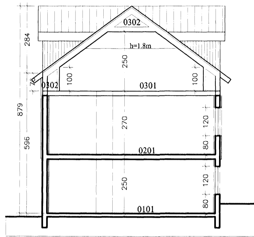
SNEIÐING a-a 1:100
