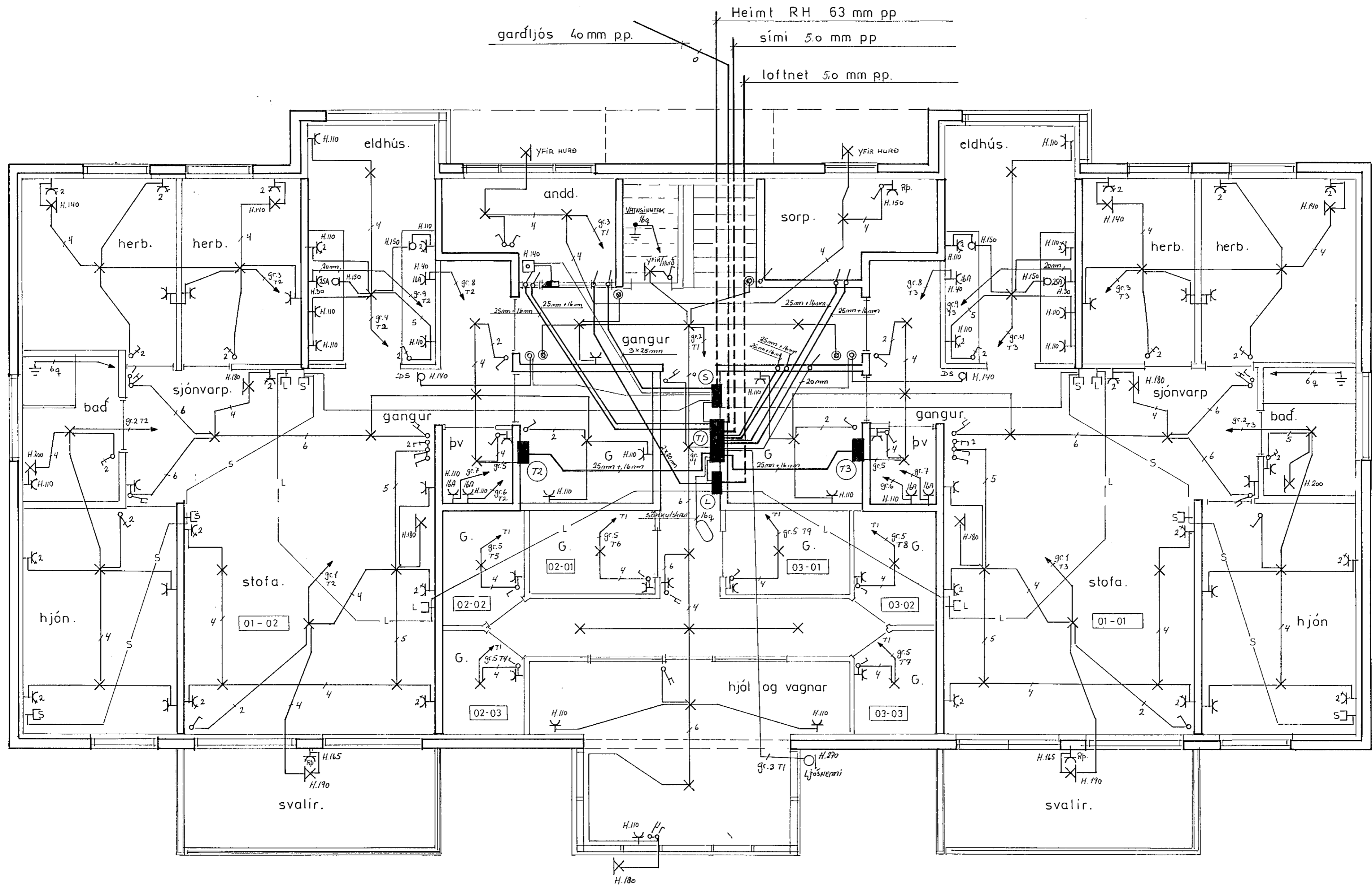
GRUNNMYND 1. HÆÐAR MÁL 1:50
