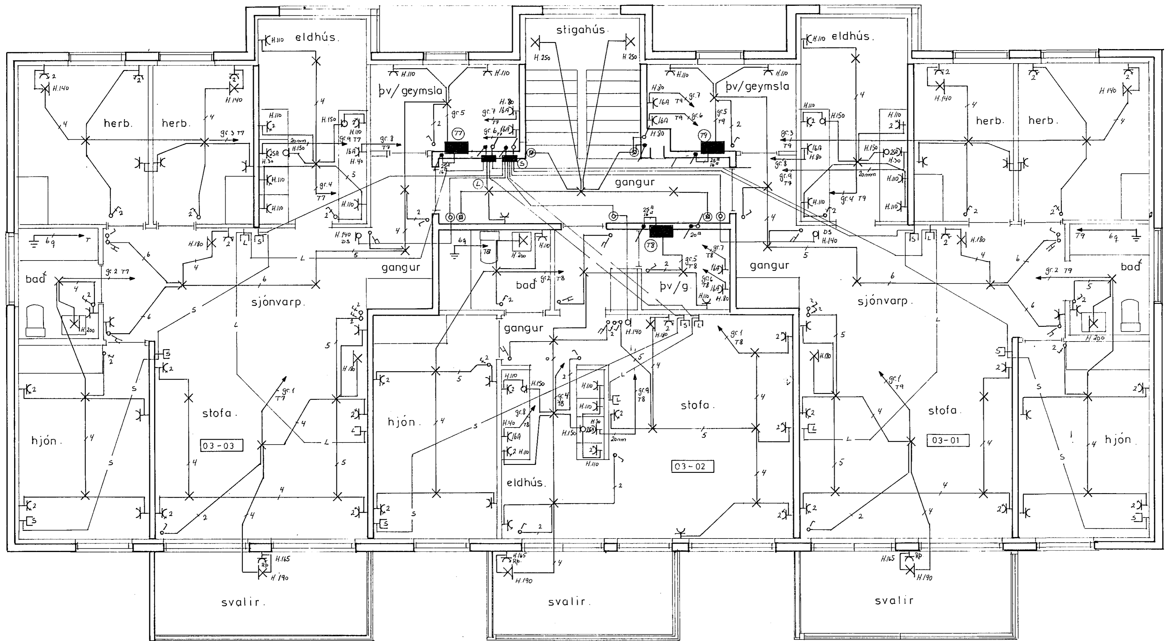
GRUNNMYND 3. HÆÐAR MÁL 1:50
