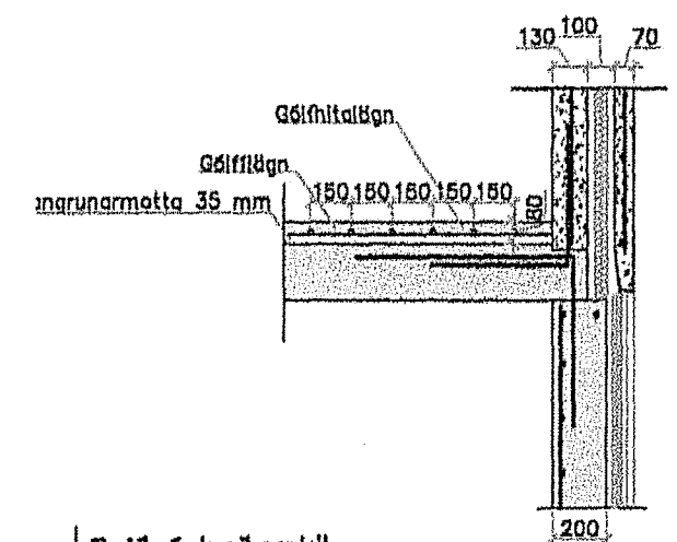
Sníð 1 hæðarskili Mkv. 10
