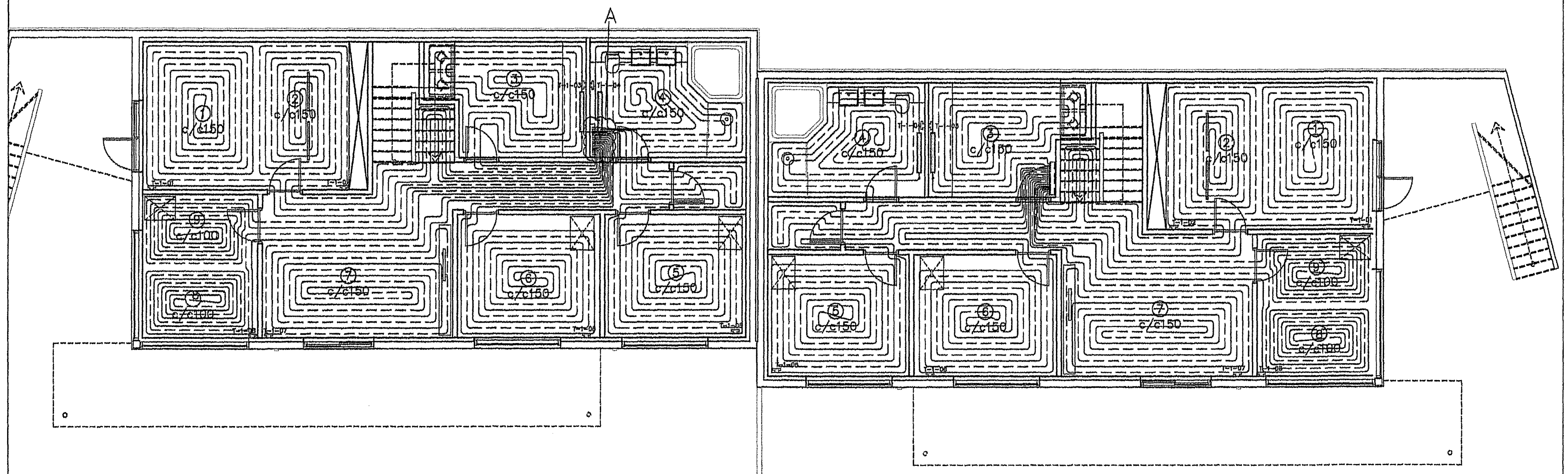
Grunnmynd 1. hæð Mkv. 1:50
