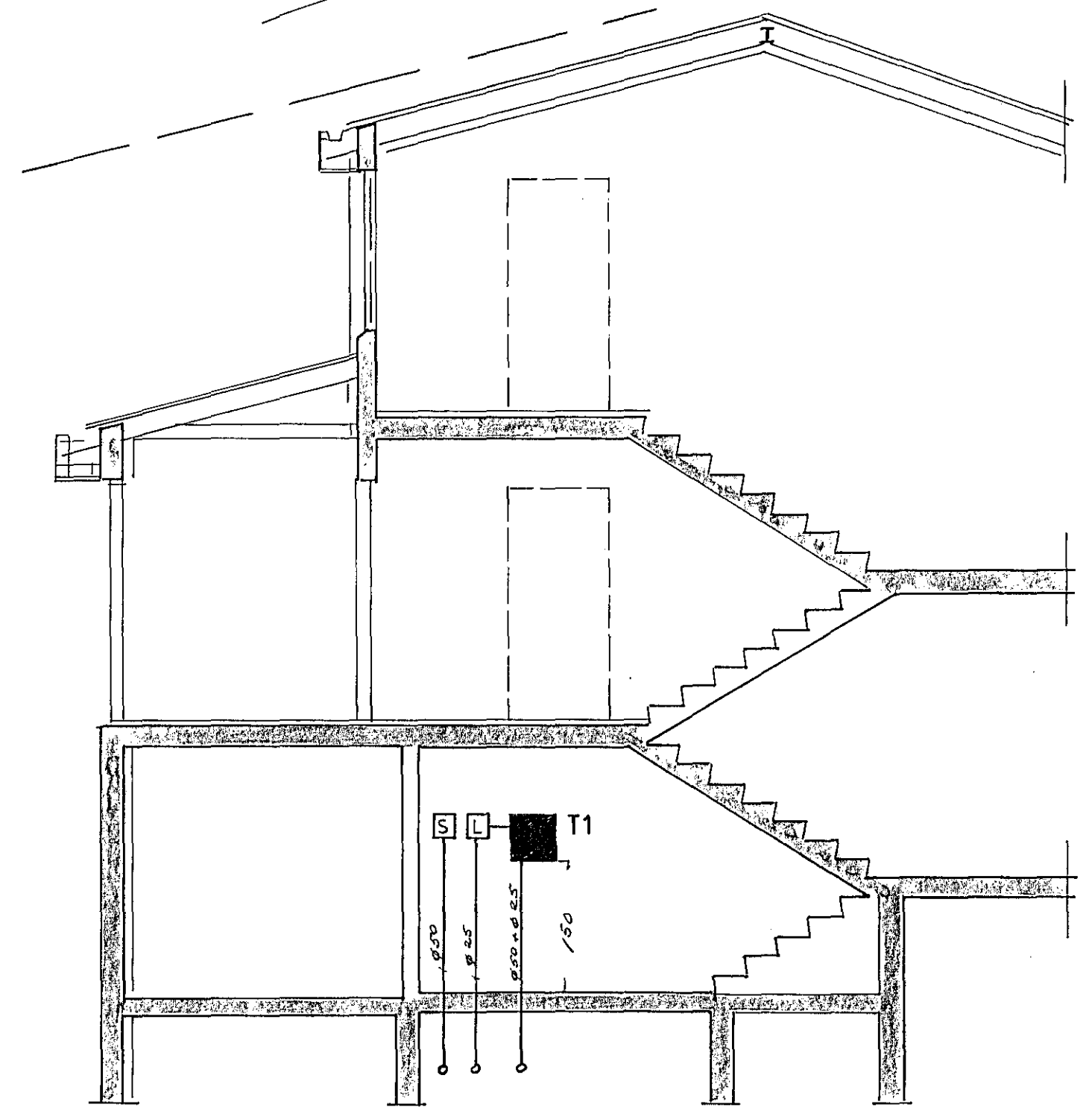
Sneiðing m. 1:50
