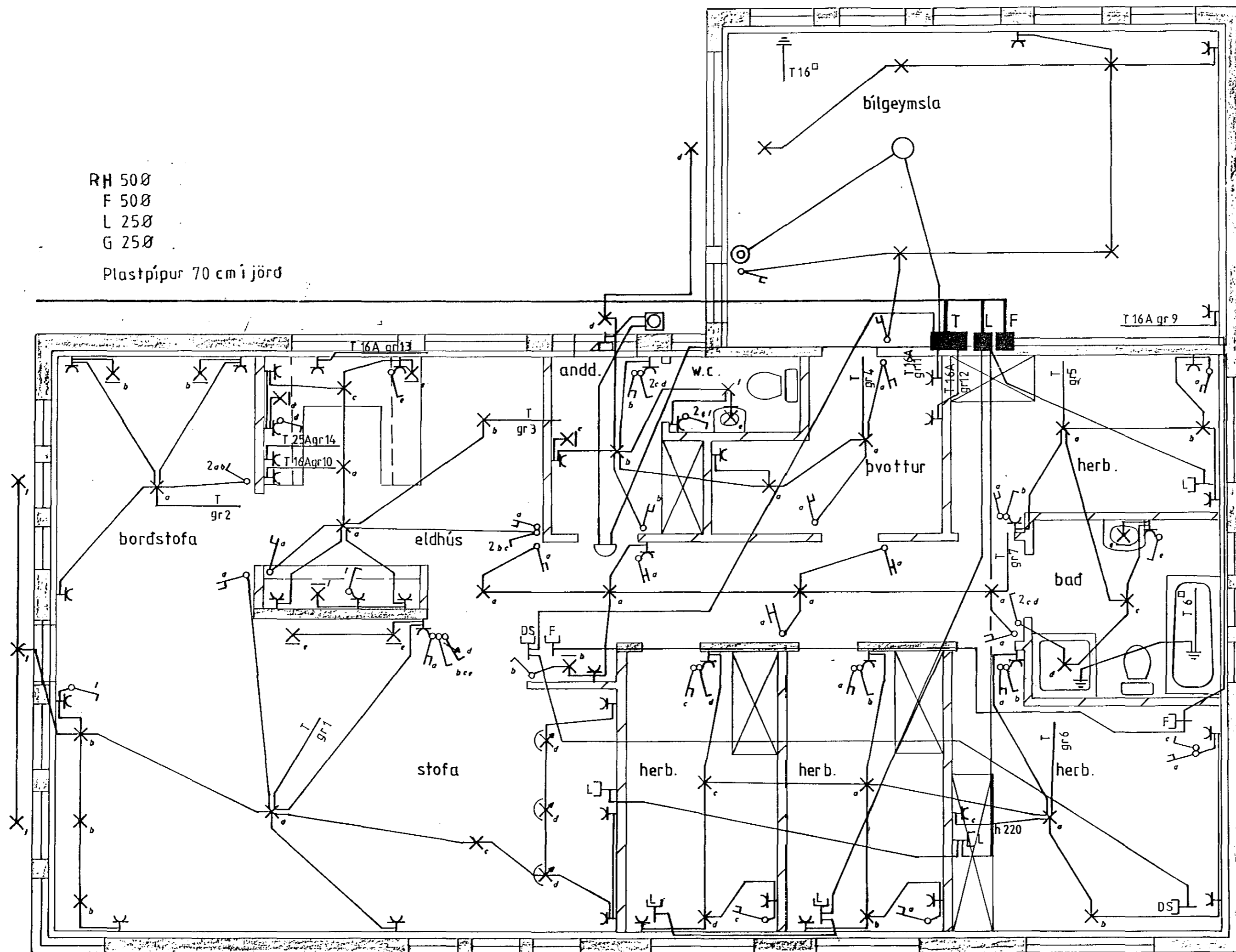
Grunnmynd mkv. 1:50
