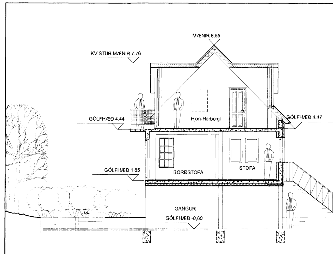
SNID A-A
