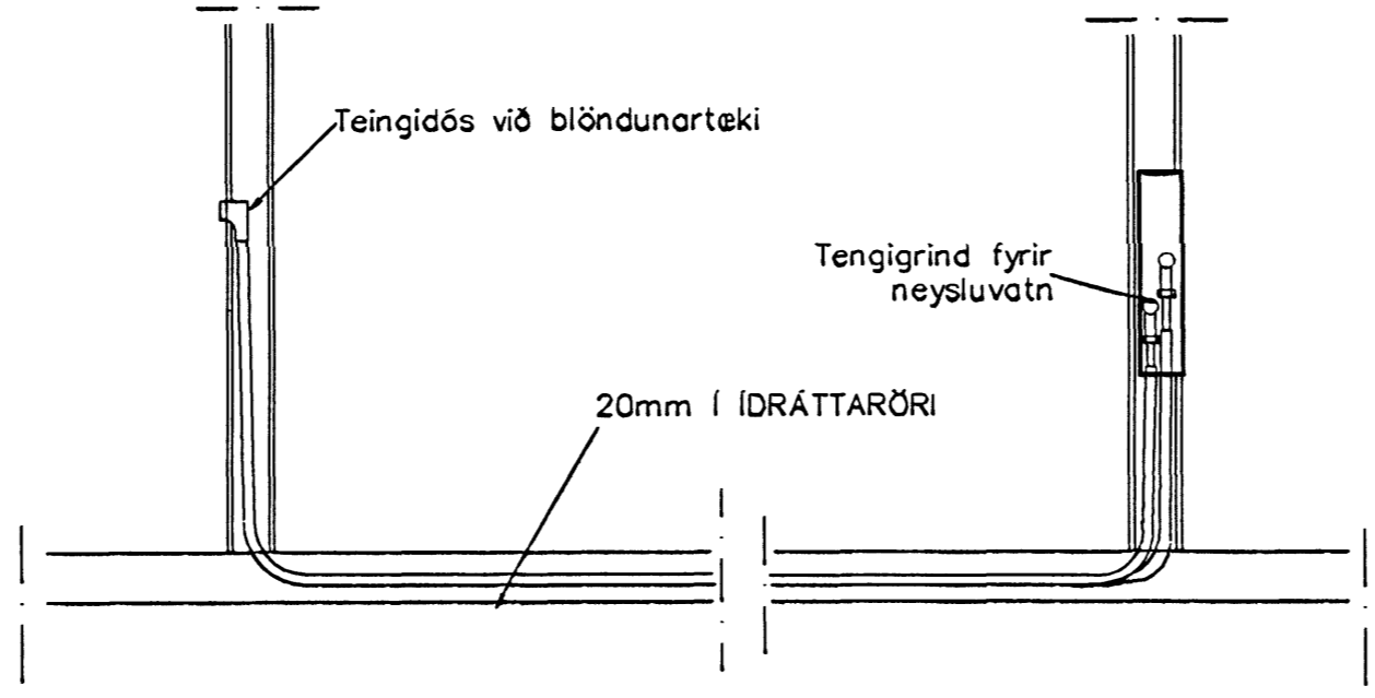
TENGING NEYSLUVATNSLAGNA 1:20
