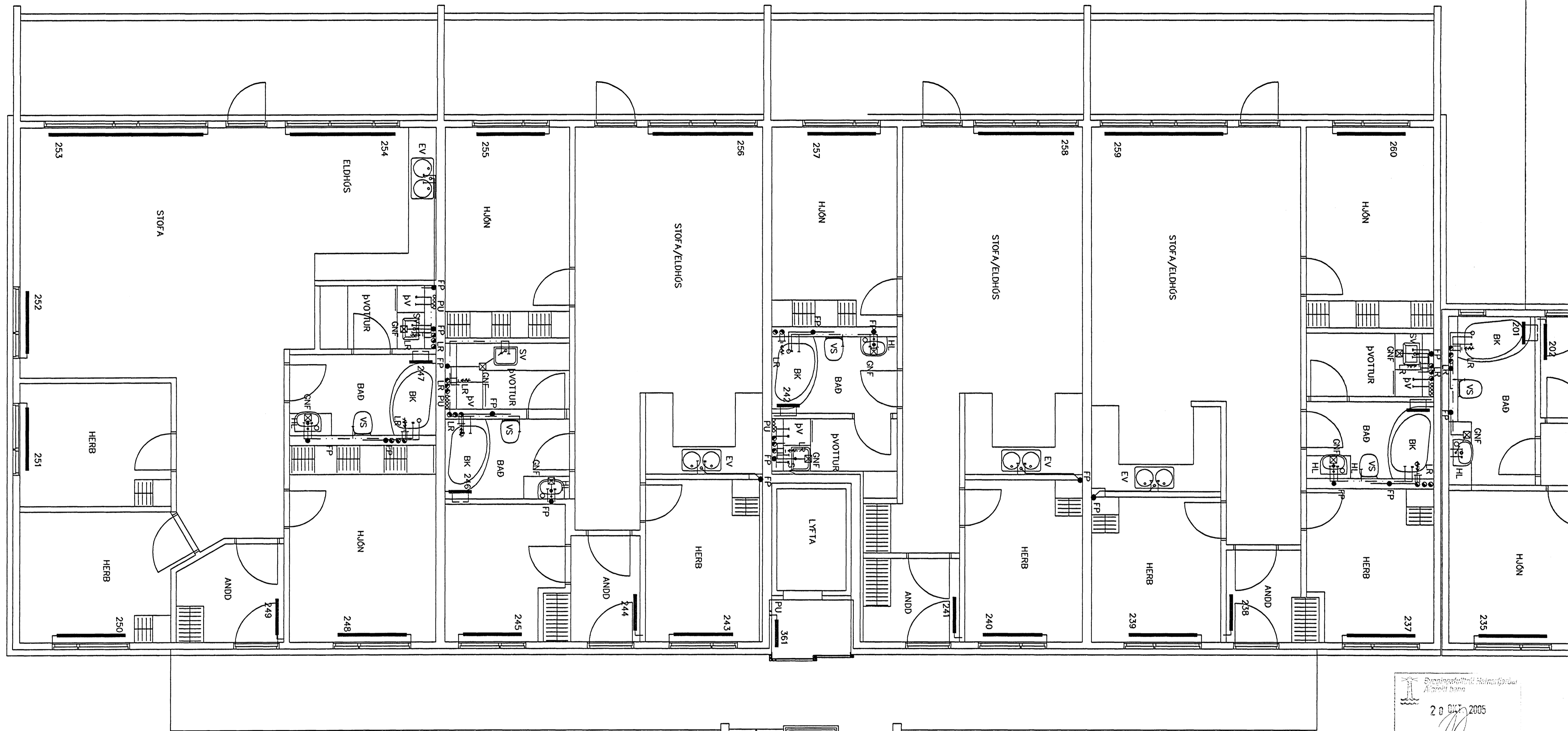
GRUNNMYND 3 HÆÐAR 1:50
