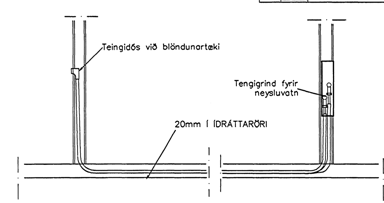
TENING NEYSLUVATNSLAGNA 1:20
