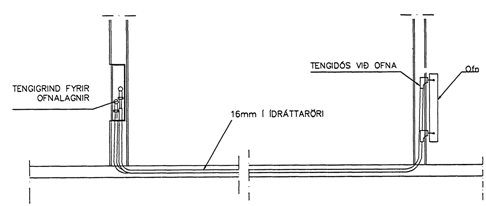
TENING OFNALAGNALAGNA 1:20
