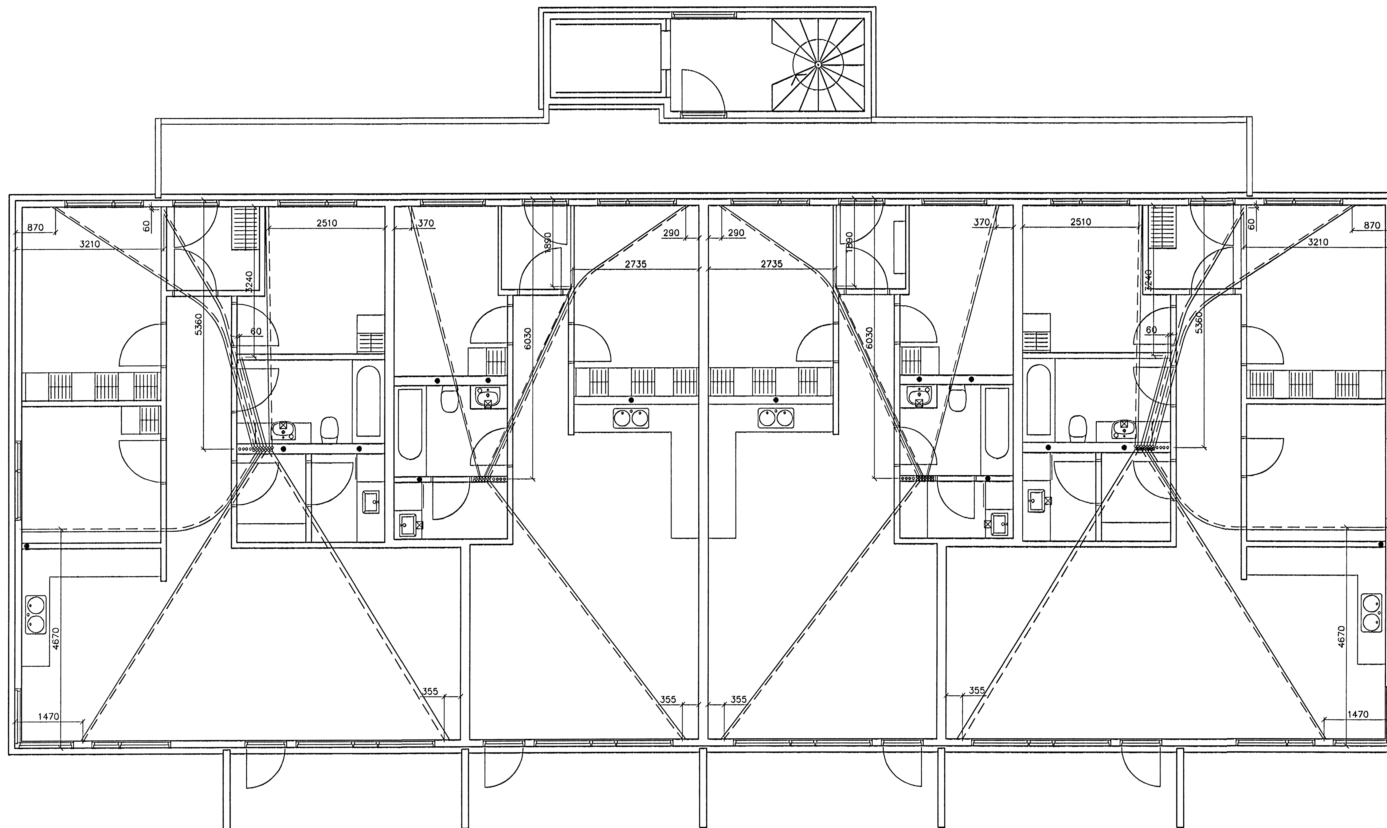
GRUNNMYND 5 HÆÐAR 1:50
