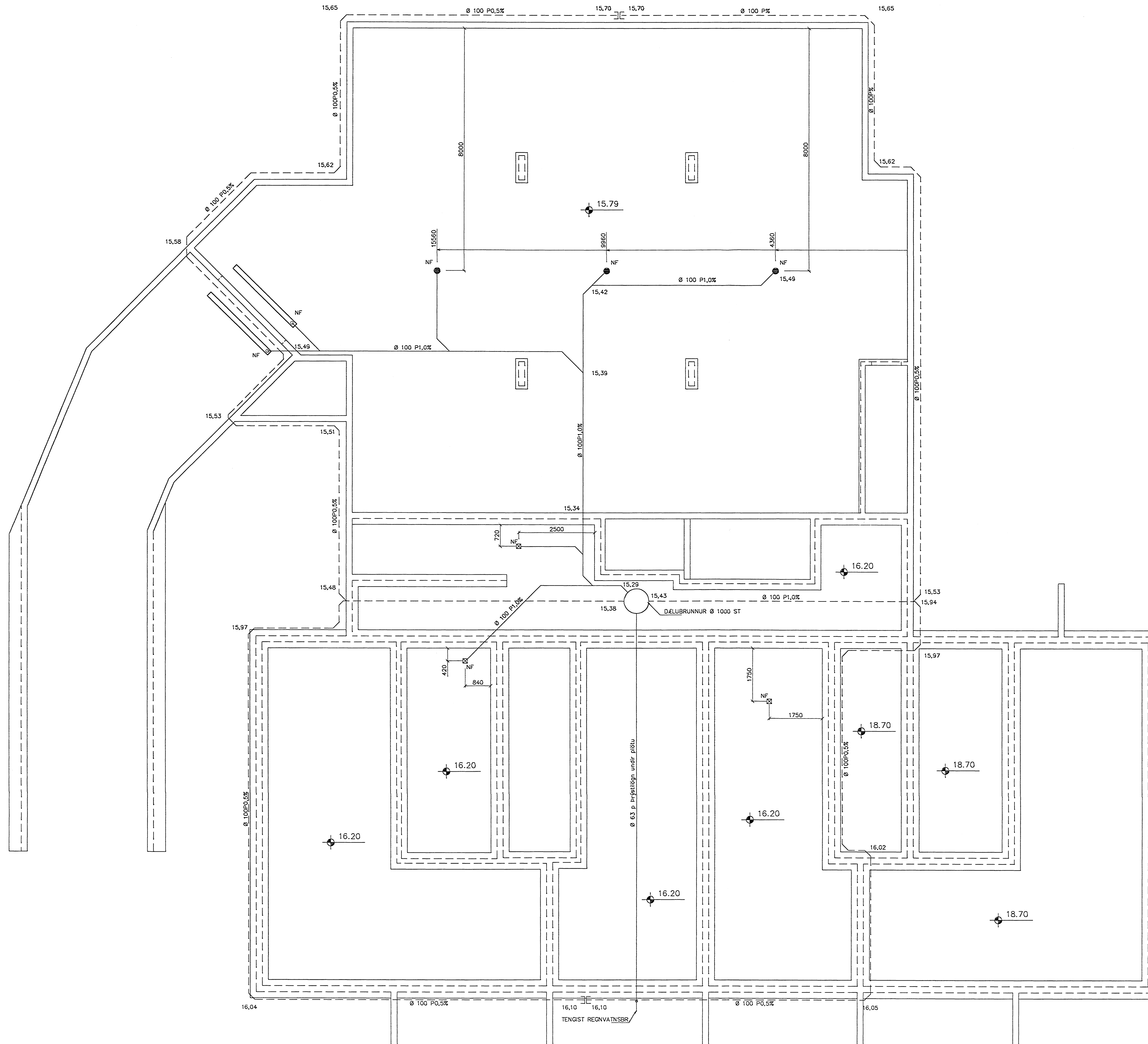
GRUNNMYND 1:50
