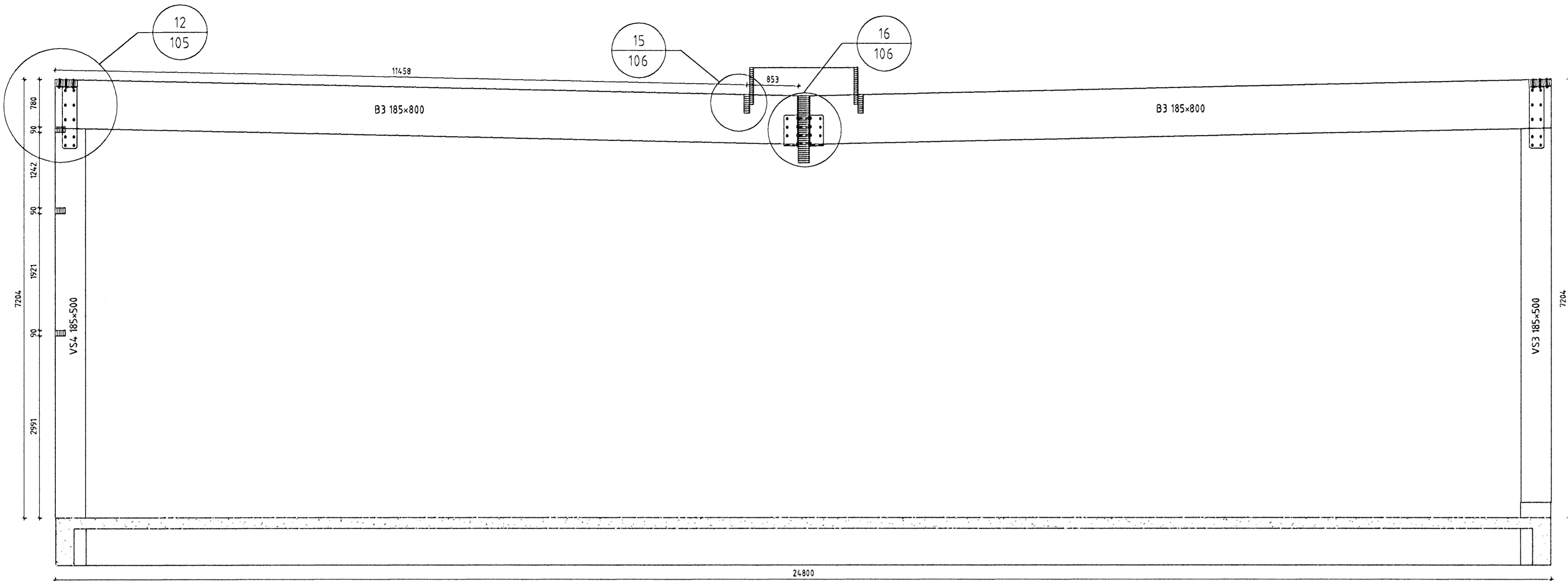
Dversnið C Mkv. 1:50 101
