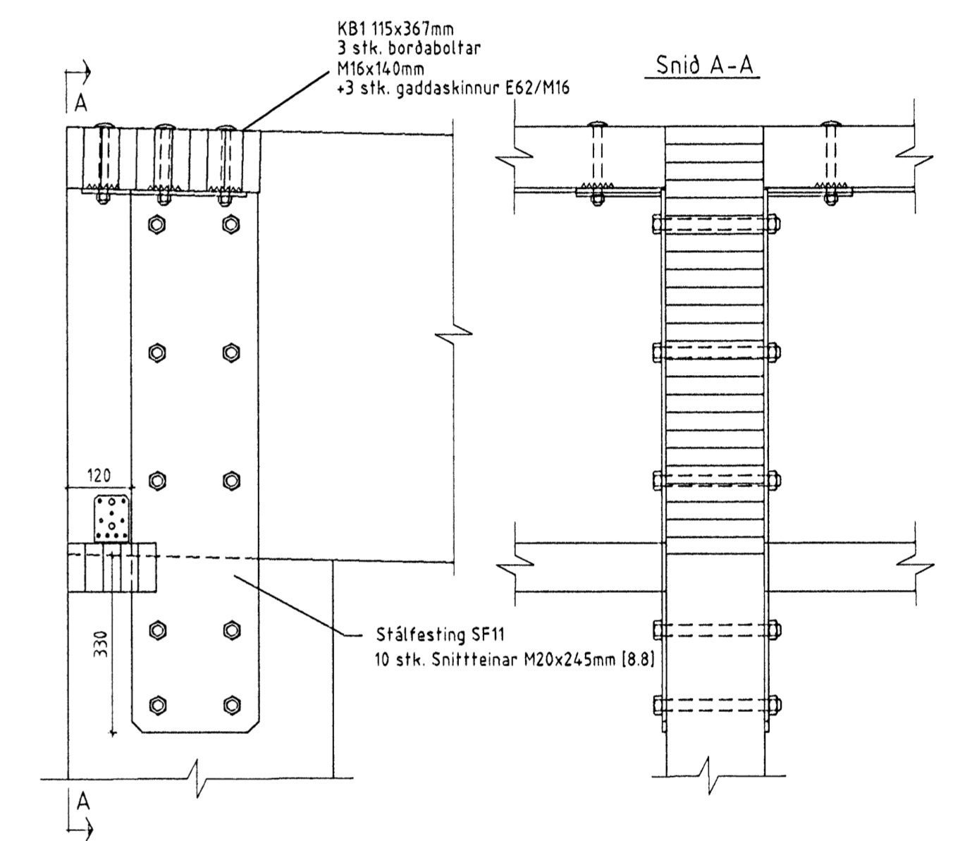
Sérmynd \frac{12}{105} Mkv. 1:10
