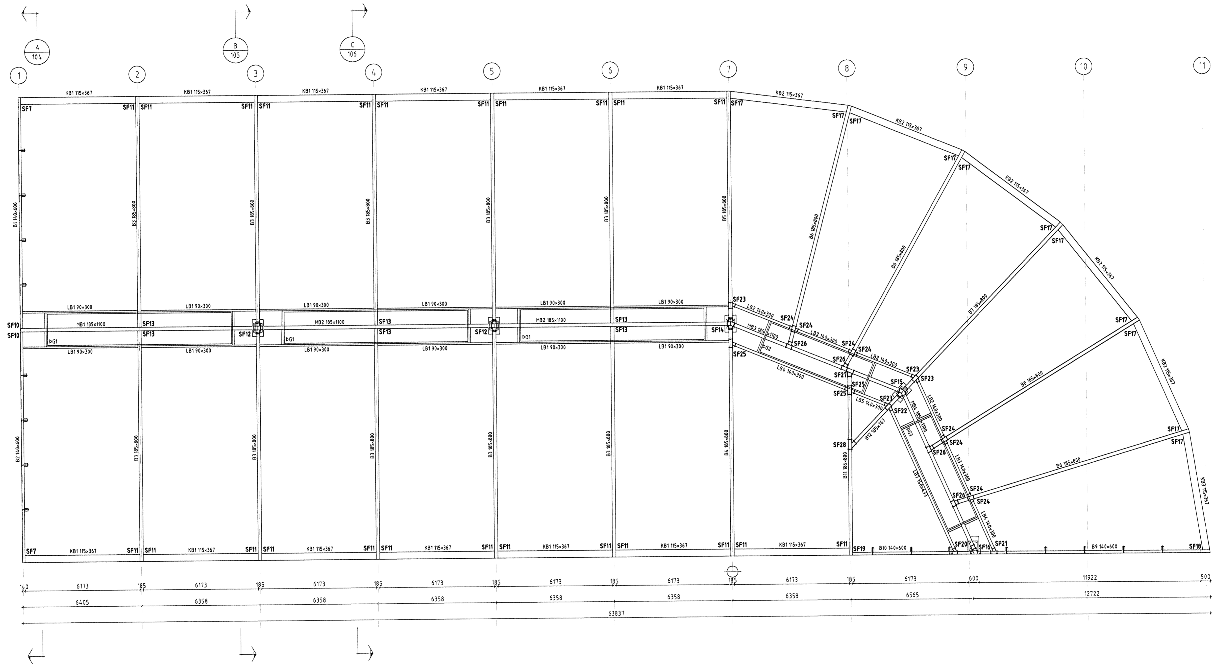
Þakmynd - Mkv.: 1:100
