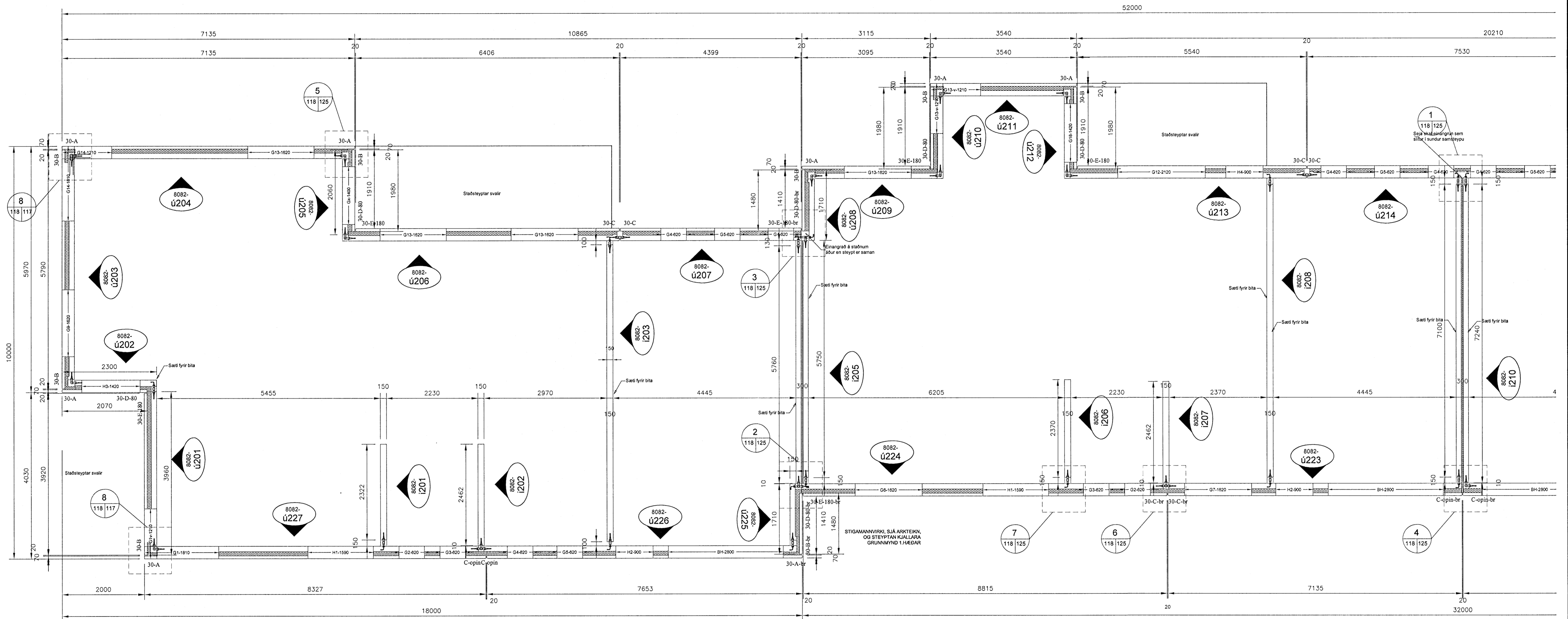
Grunnmynd - veggeininga - 2 hæð 1:50
