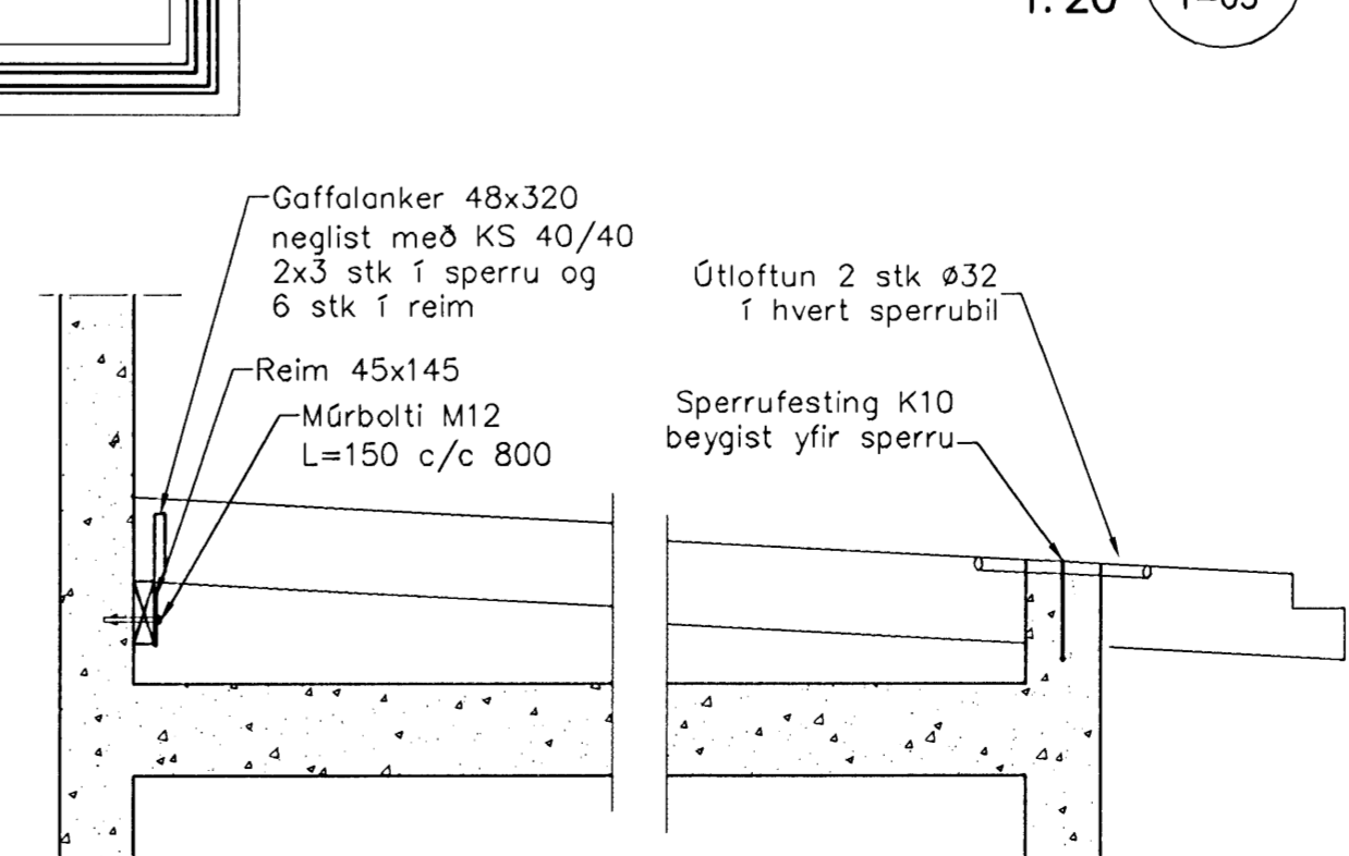
Snið 4 1:20 1-05
