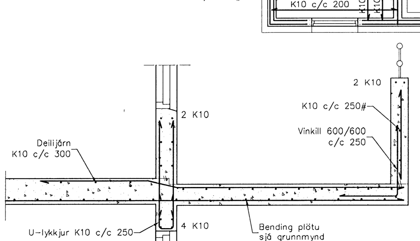
Snið 3 1:20 1-05
