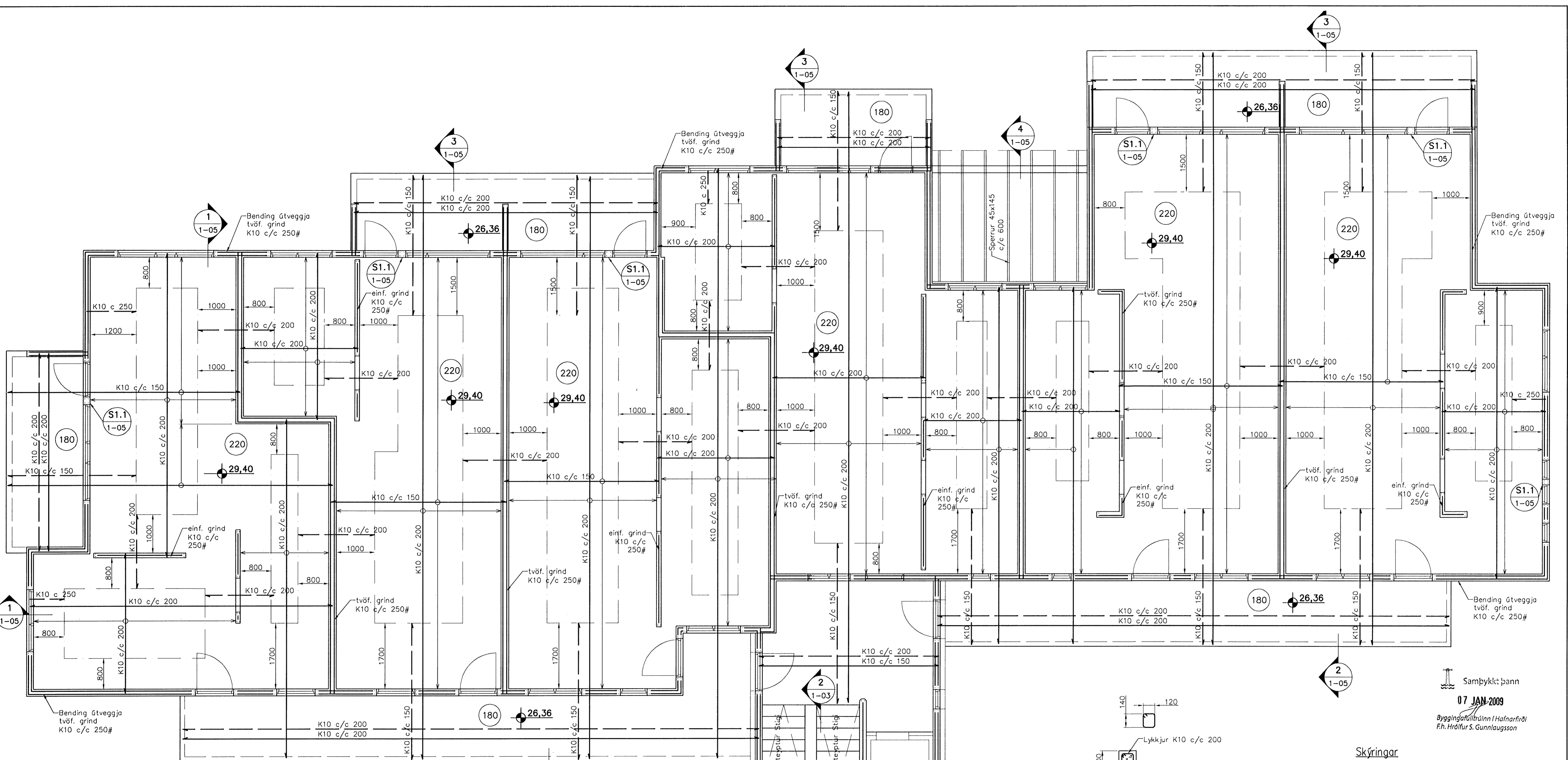
Veggir 2. hæð, Plata yfir 2. hæð, Grunnmynd, 1:50
