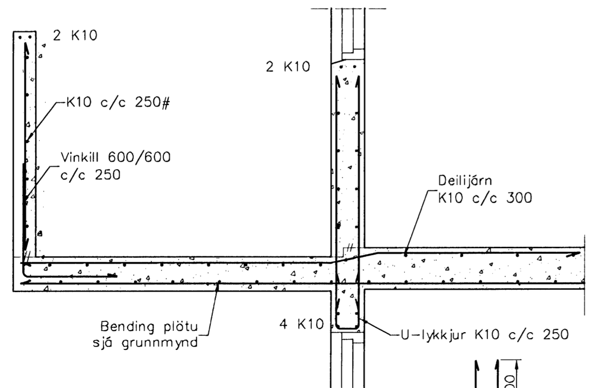
Snið 2 1:20 1-05
