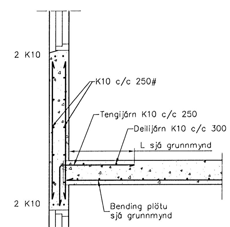
Snið 1 1:20 1-05
