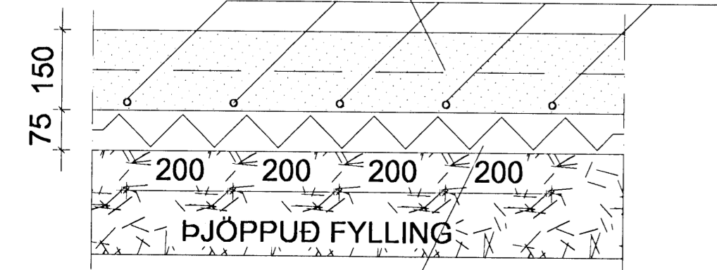
SNID Í GÓLFPLÖTU Í SKRIFSTOFUM OG ANDDYRI
