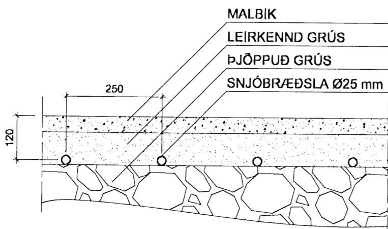
SNID Í PLAN MKV. 1:10
