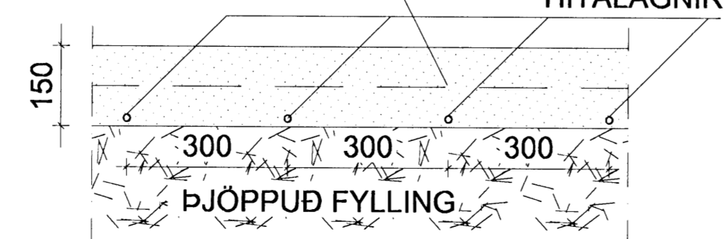
SNID Í GÓLFPLÖTU Í RYÐFRÍUM SAL
