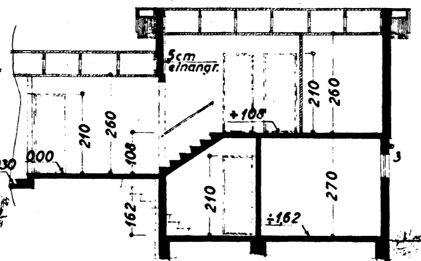
Snið: B-B
