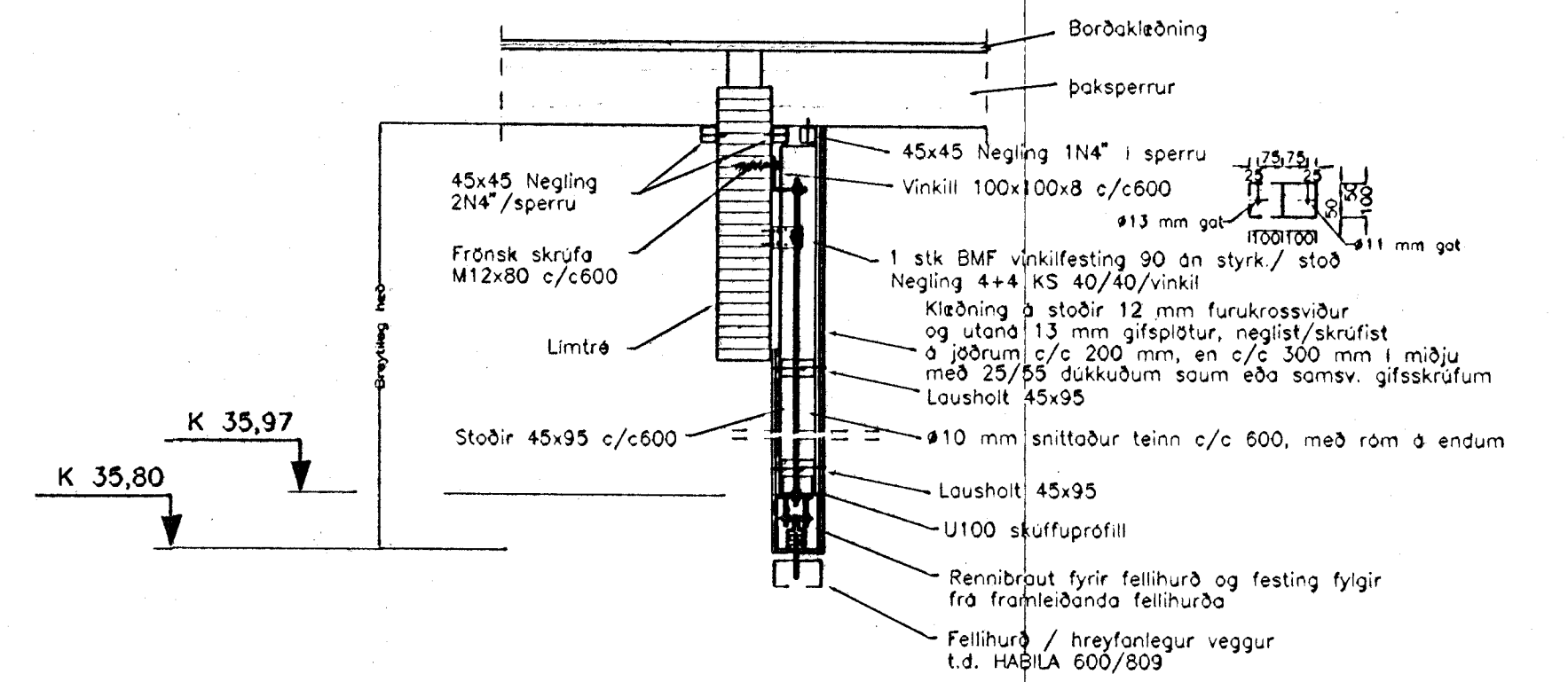
F28 SNID, Mkv. 1:20
