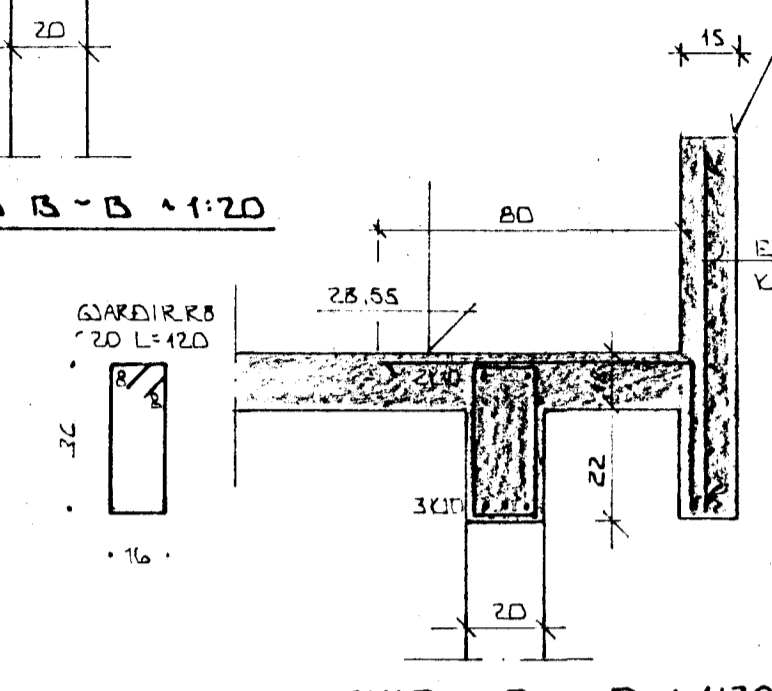
SNID D - D ~ 1:20
