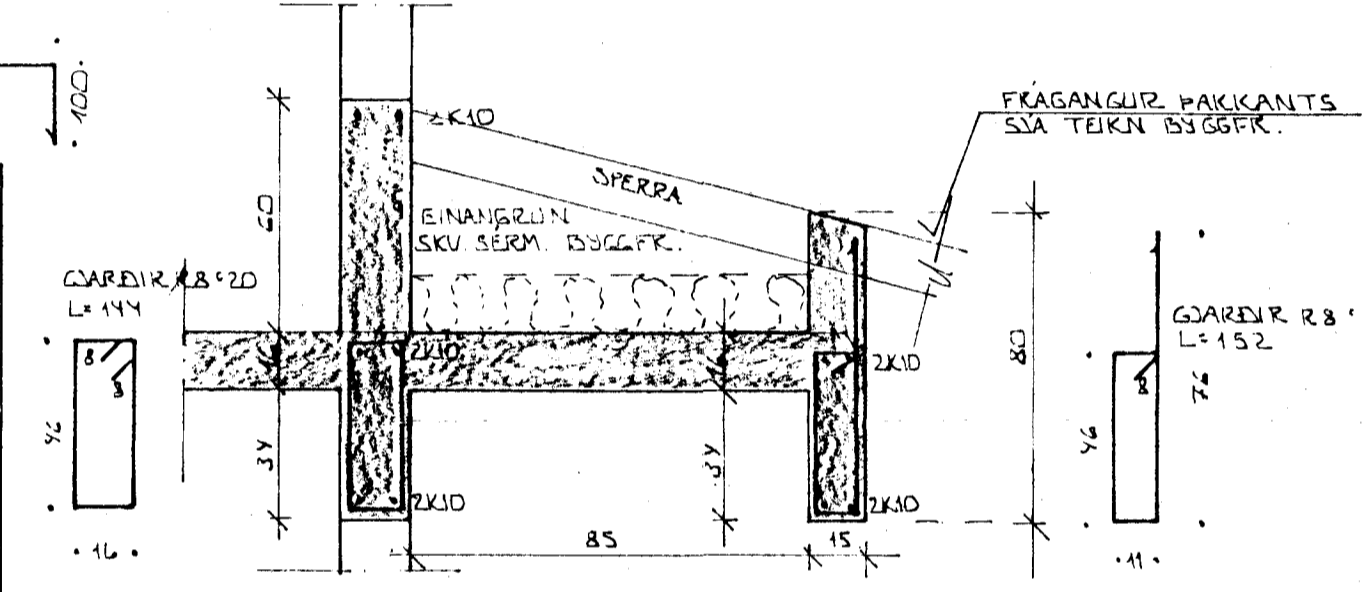
SNID C - C ~ 1:20
