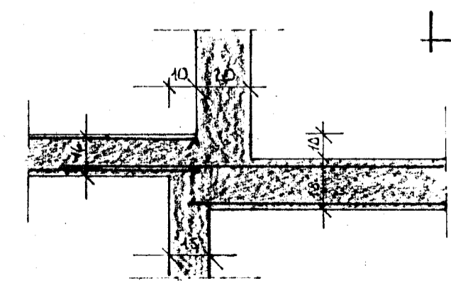
SNID E - E ~ 1:20
