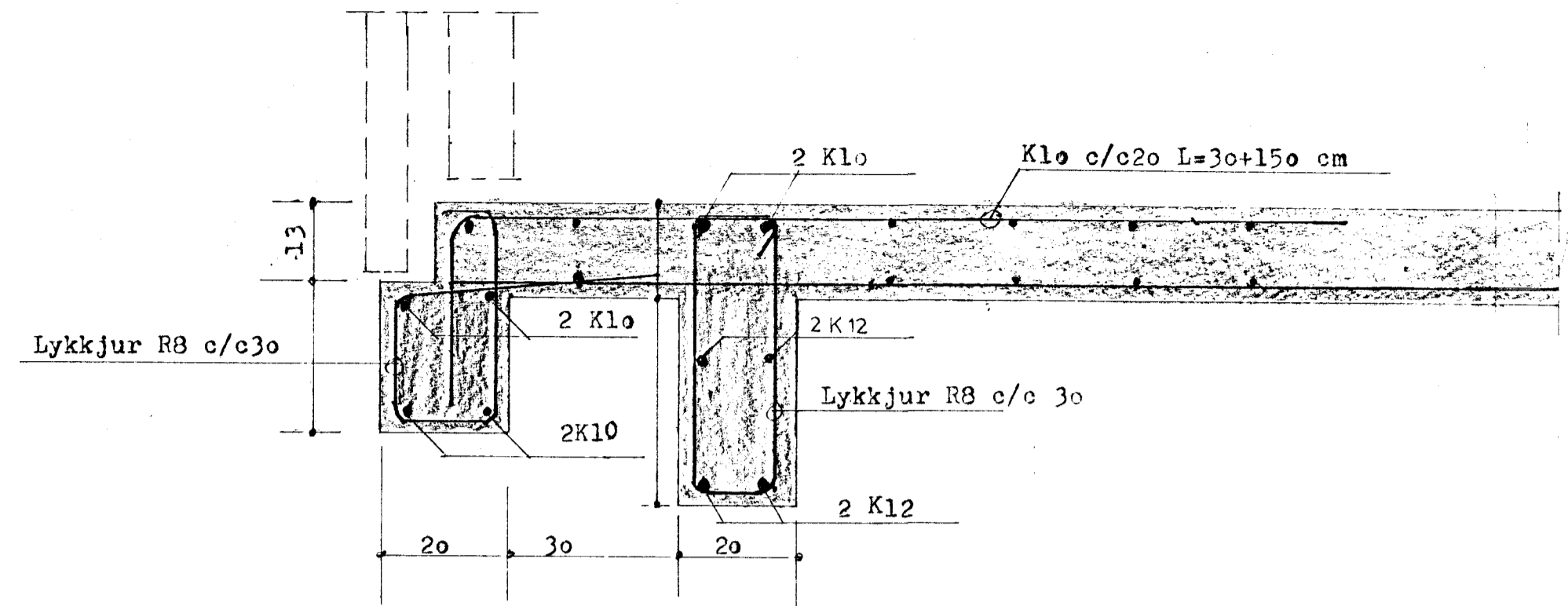
Snið A-A. M= 1:10
