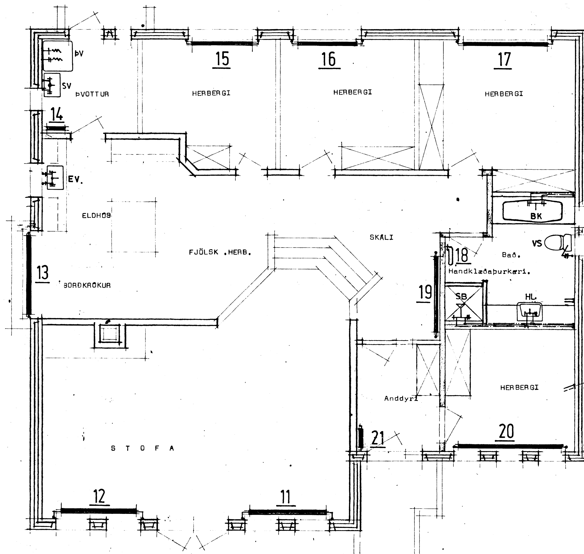
Grunnmynd Mk 1:50
