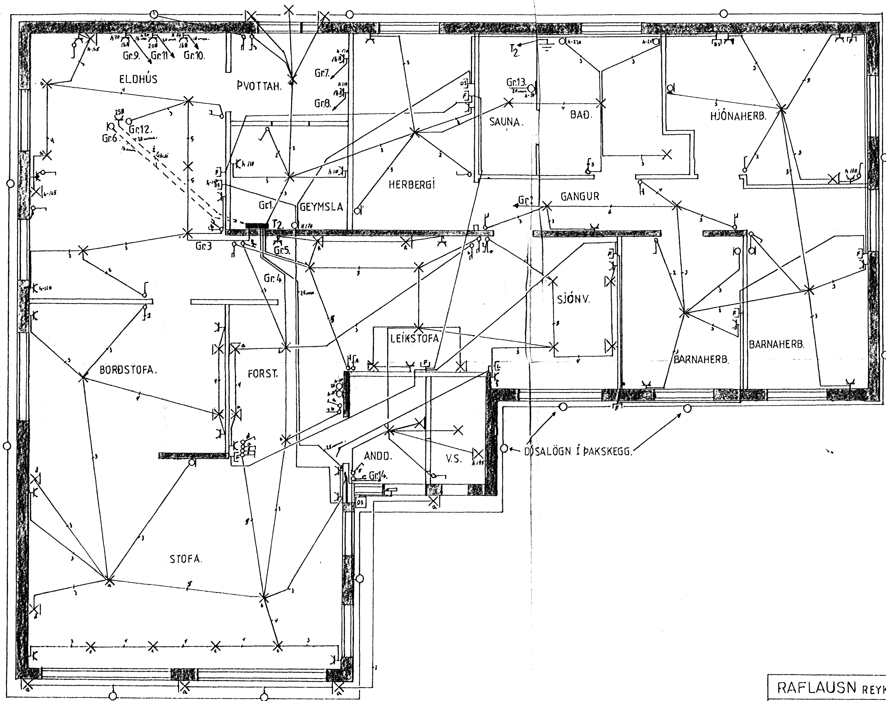
GRUNNMYND RAFLAGNA 1 HÆÐ. 1:50.
