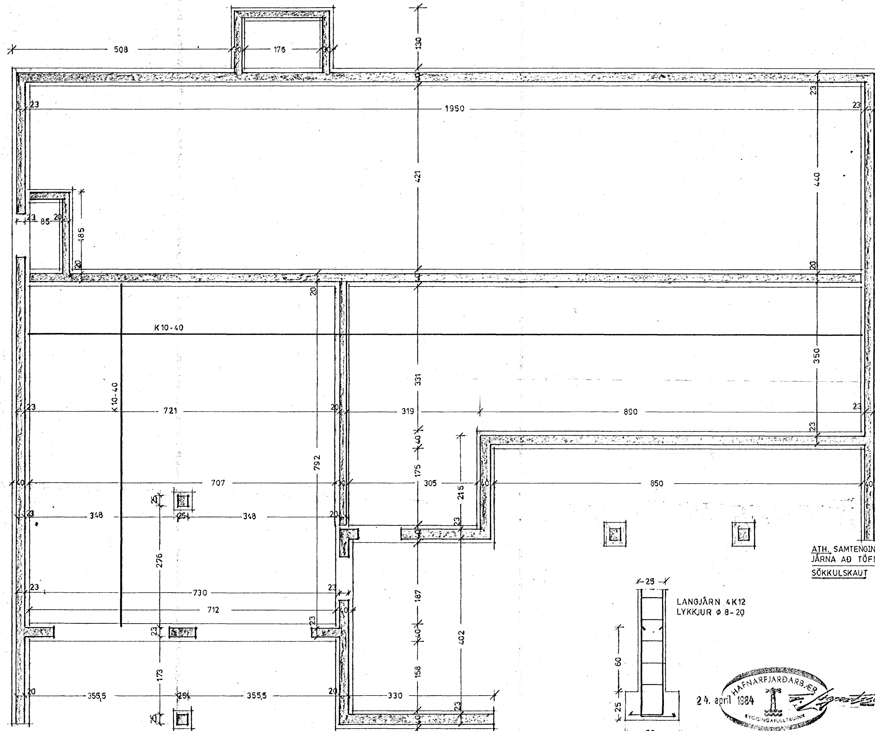
GRUNNMYND. UNDIRSTÖÐUR. 1:50
