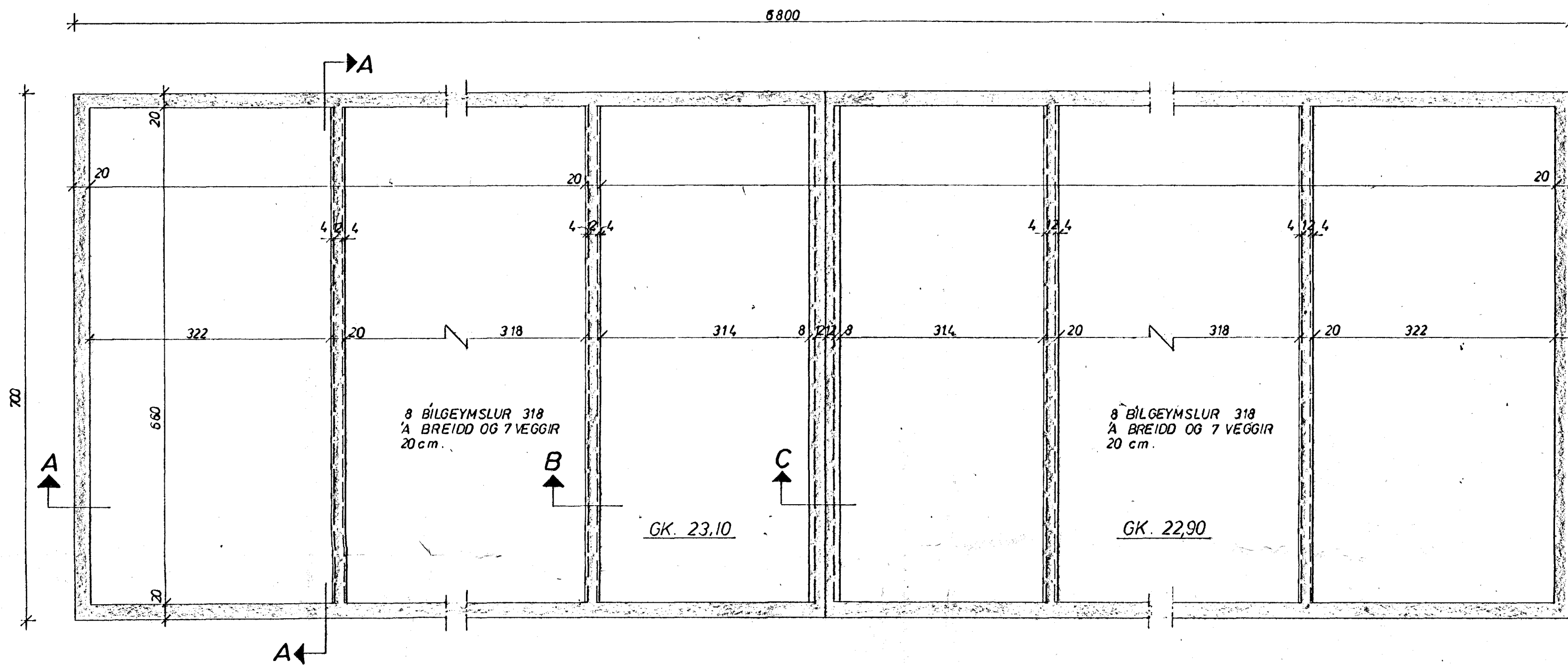
GRUNNMYND 1:50
