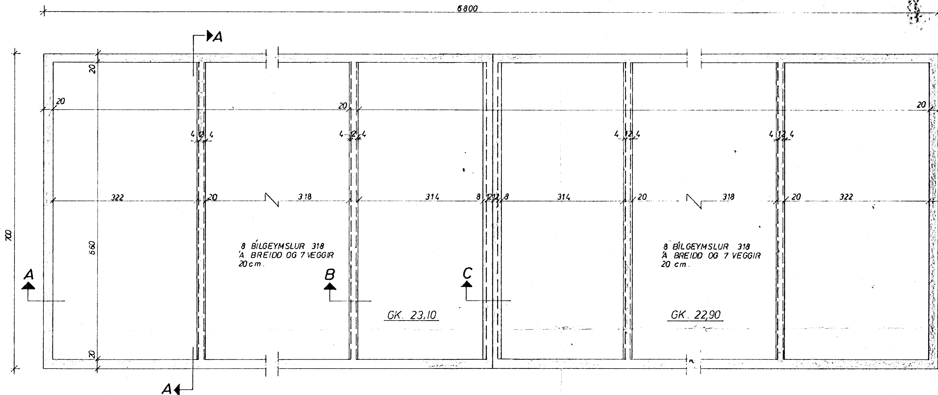
GRUNNMYND 1:50
