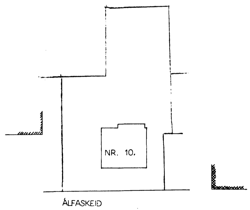
AFSTÖÐUMYND 1:500
