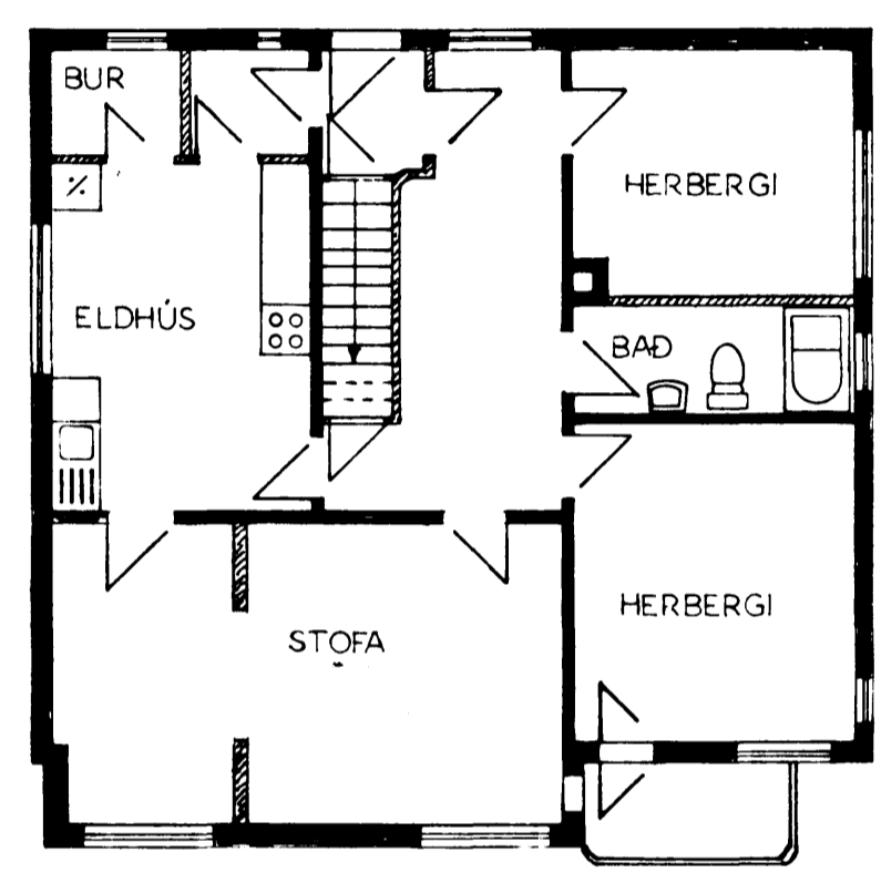
1. HÆÐ
