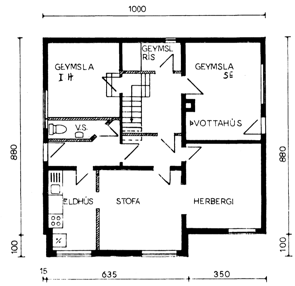
KJALLARI
