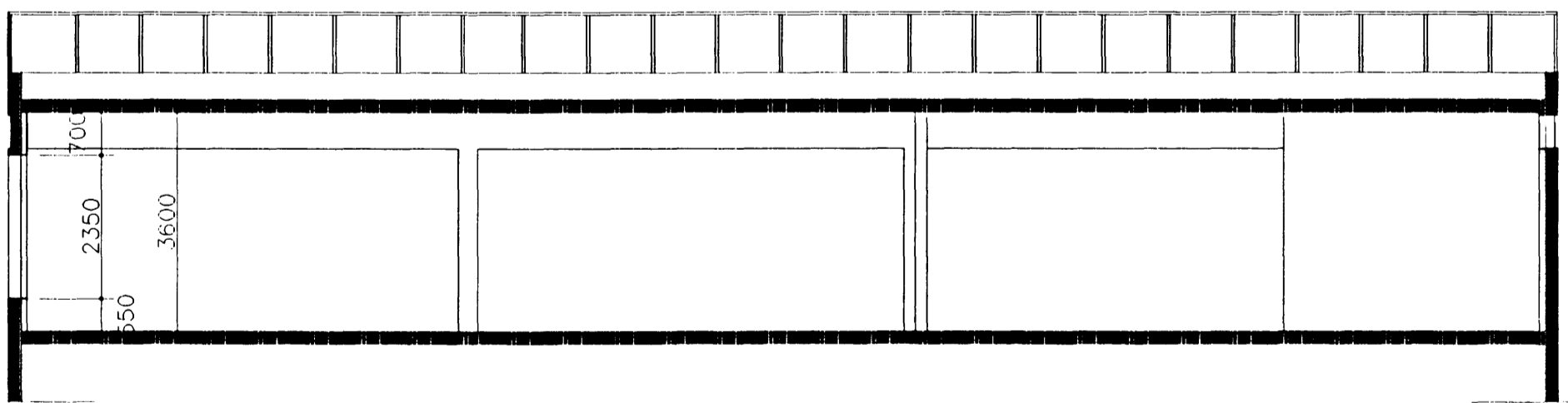
SKURÐUR A-A 1/100
