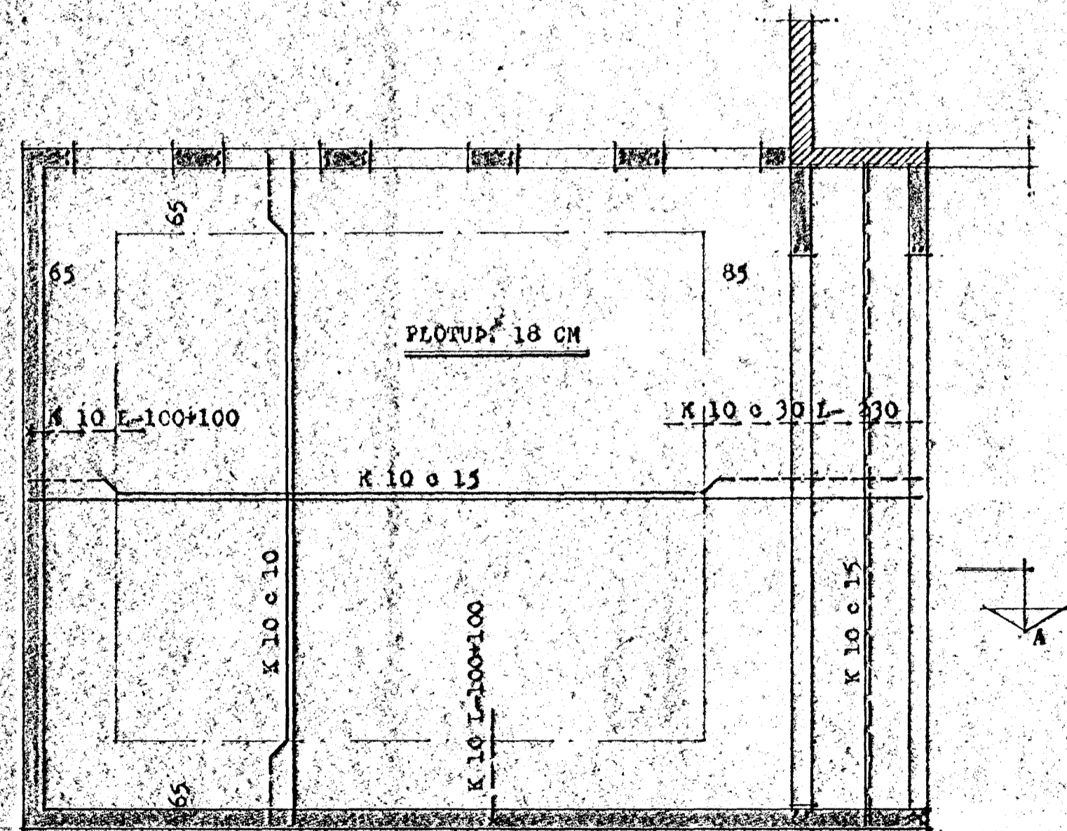
GRUNNMUND 1:50
