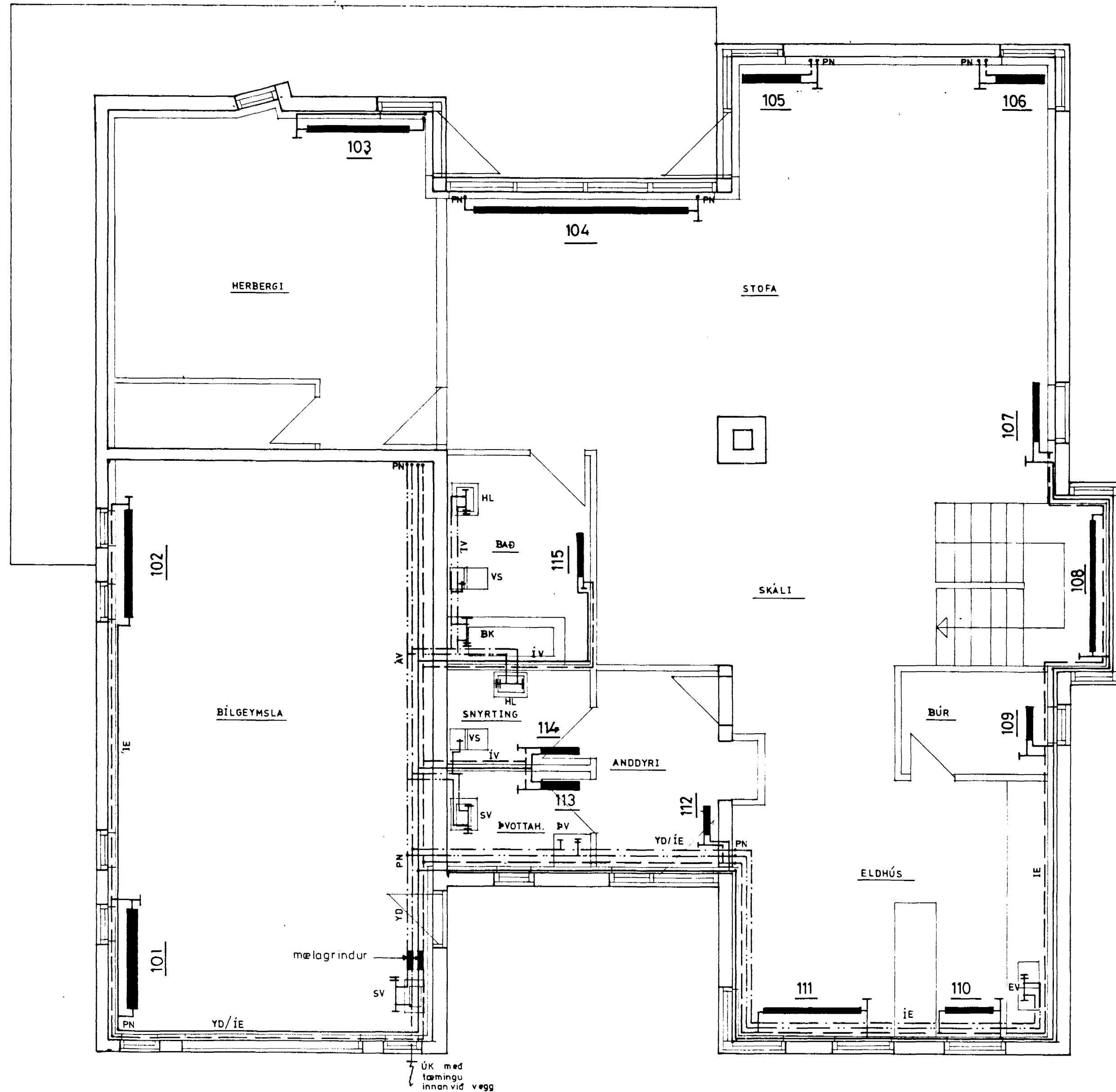
Grunnmynd neysluvatns og hitalagna á 1.hæð. mkv. 1:50
