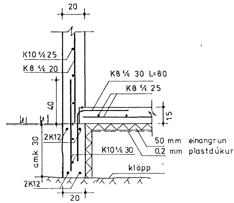
SNID 1-1 mkv. 1:20
