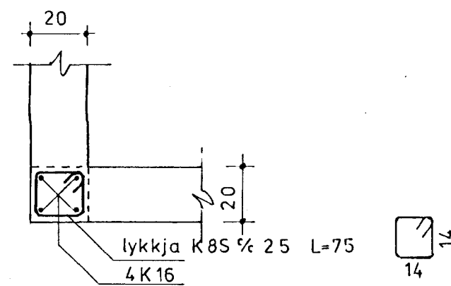
SÚLA S1 mkv. 1:20
