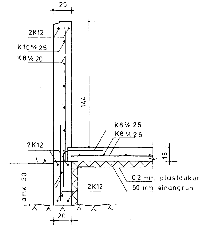
SNID 5-5 mkv. 1:20
