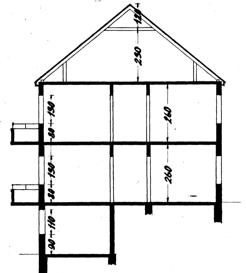
Þverskurður
