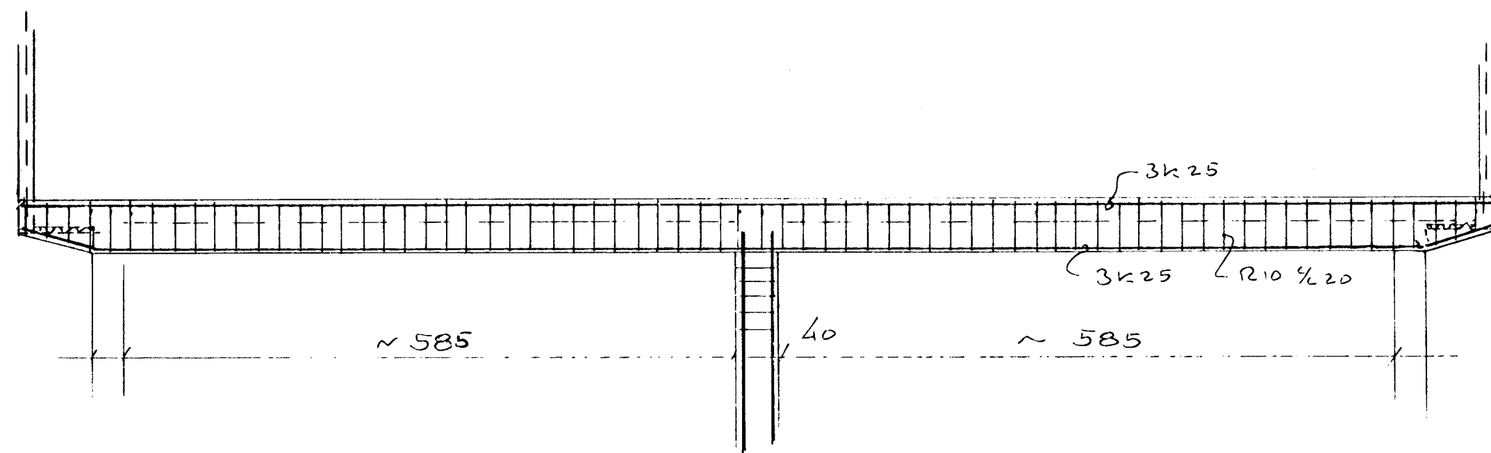
VEGGBITI 1:50
