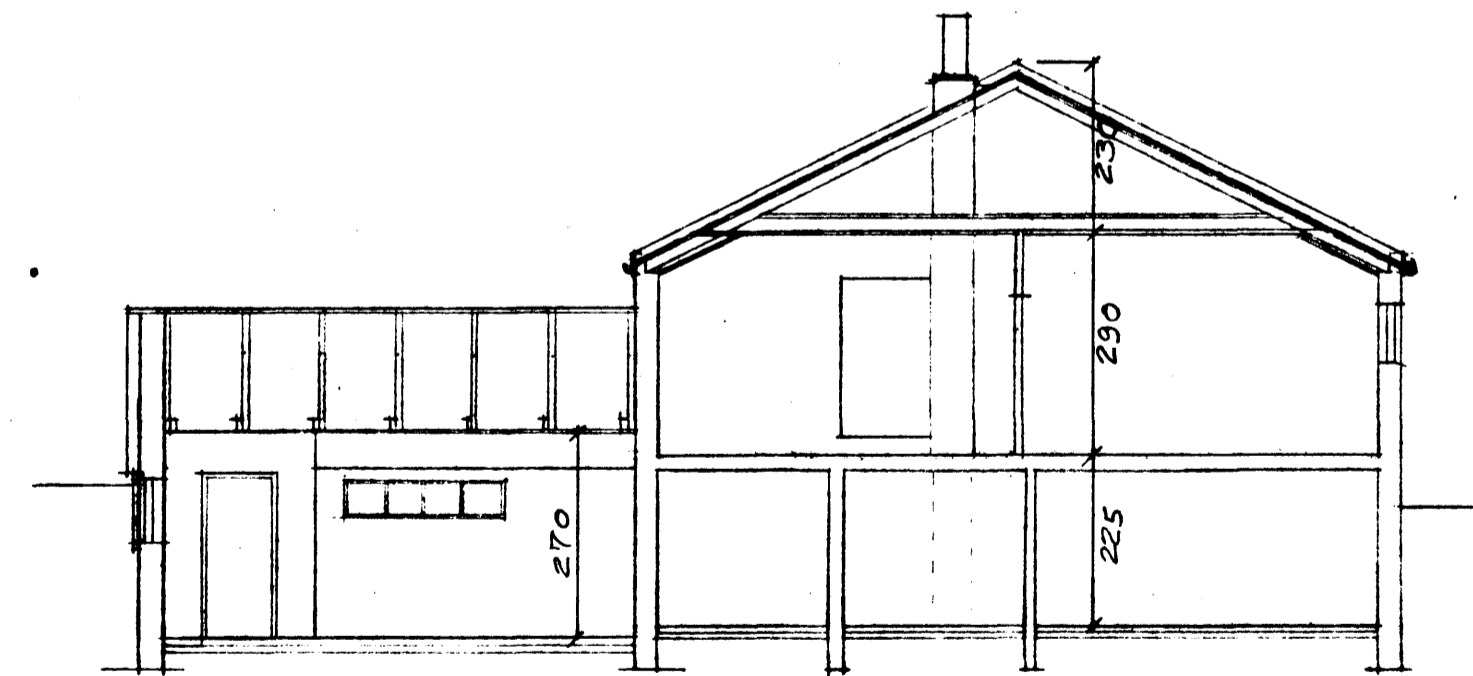
SNÍÐ A-A 1:100
