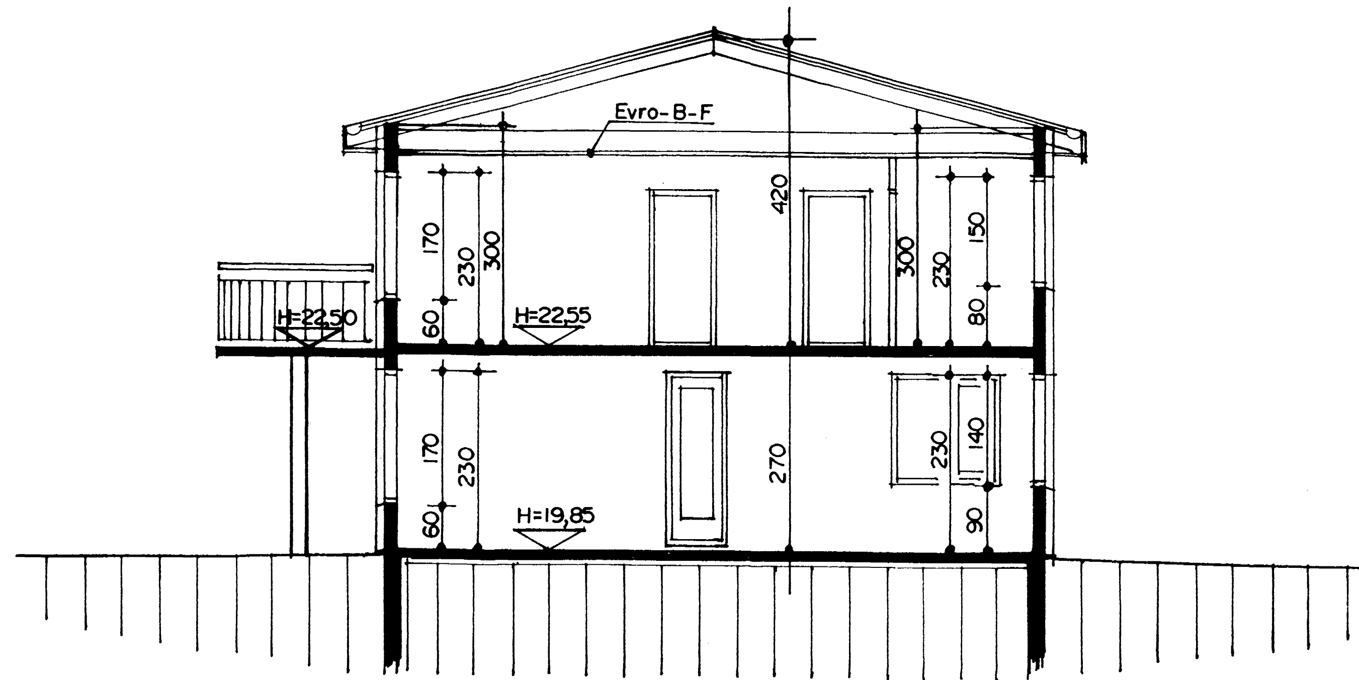
SNIÐ A-A MKV. 1:50.
