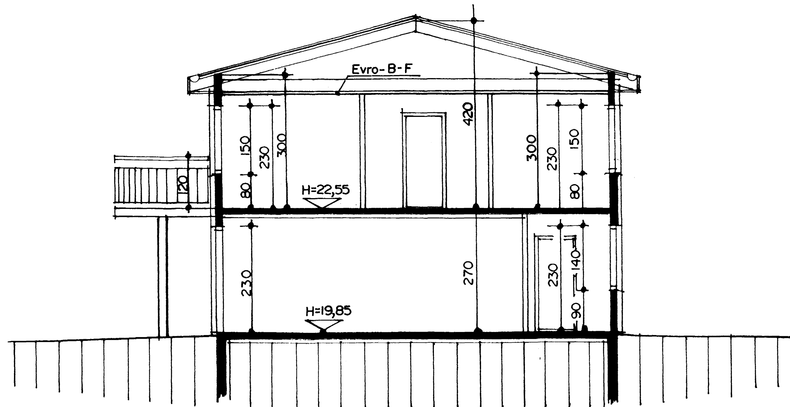
SNIÐ B-B MKV. 1:50.
