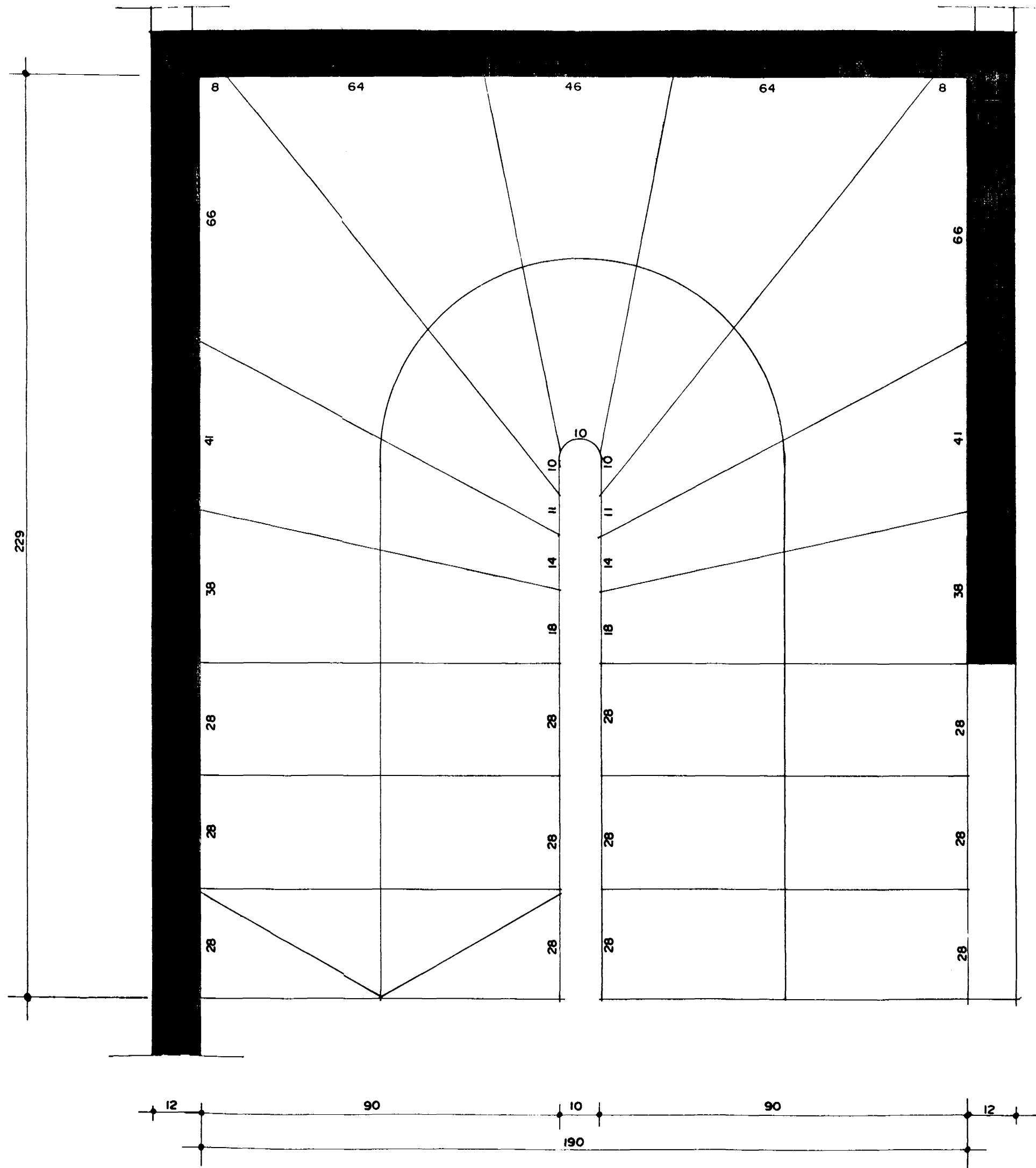
GRUNNMYND STIGI MKV. 1:10.
